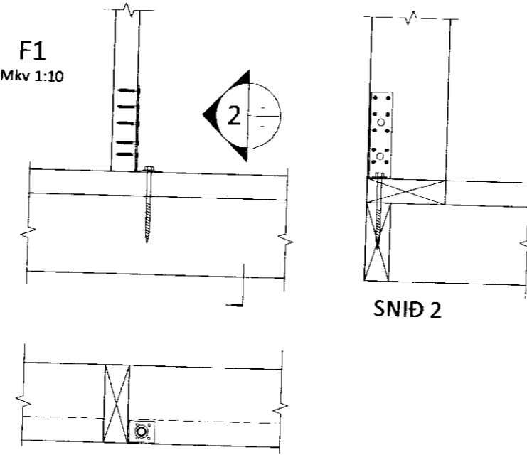
1 stk. BMF 160x50x40x3 vinkill. Festist með 5 stk. KS 40/40 í stoðir og 1 stk. M10x140 FRÖNSKUM SKRÚFUM Í GÓLFABITA, FYRIR HVERN VINKIL.
