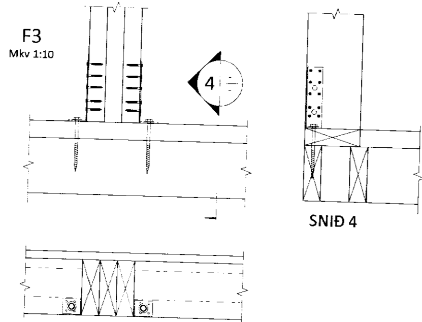
2 stk. BMF 160x50x40x3 vinklar. Festist með 10 stk. KS 40/40 í stoðir og 1 stk. M10x140 FRÖNSKUM SKRÚFUM Í GÓLFABITA, FYRIR HVERN VINKIL.
