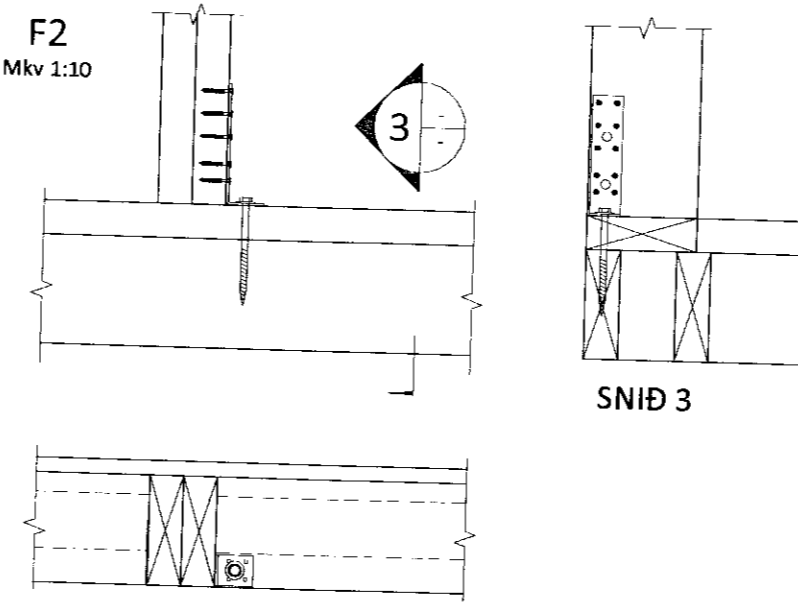
1 stk. BMF 160x50x40x3 vinkill. Festist með 10 stk. KS 40/40 í stoðir og 1 stk. M10x140 FRÖNSKUM SKRÚFUM Í GÓLFABITA, FYRIR HVERN VINKIL.
