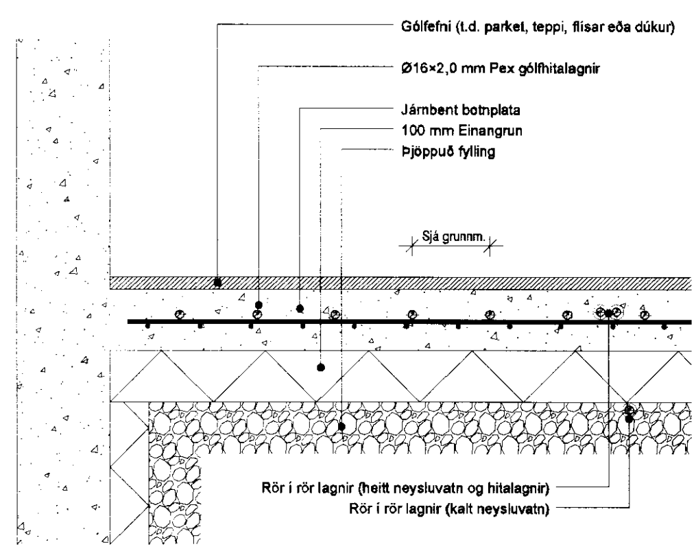
KENNISNIÐ GÓLFHITA 1:10
