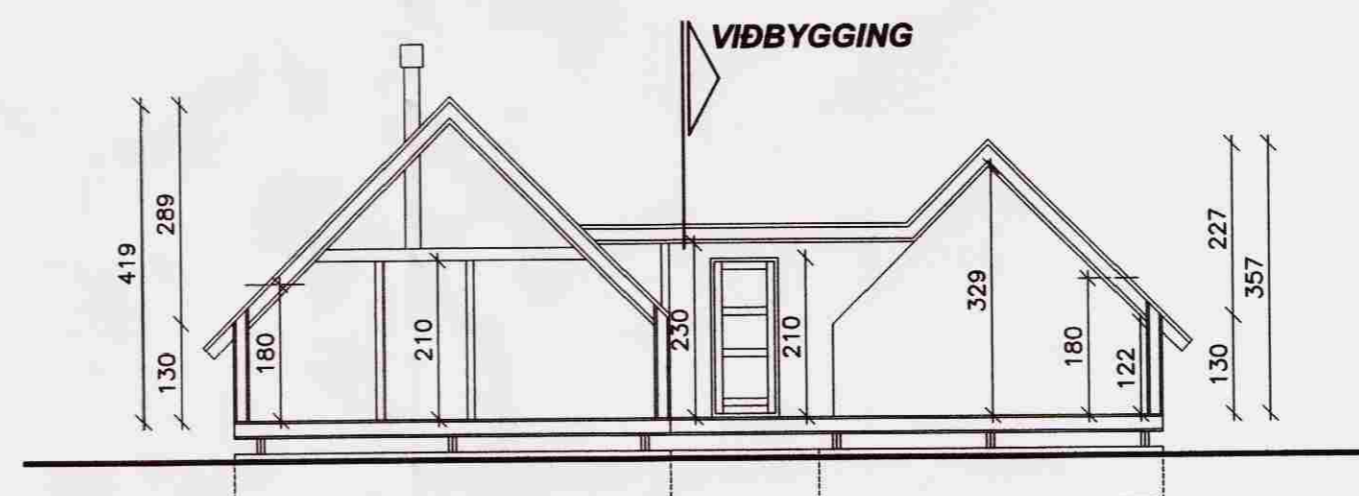
SKURÐUR A
