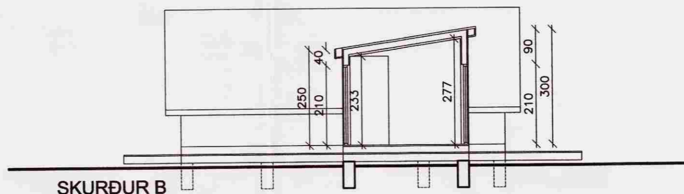
SKURÐUR B
