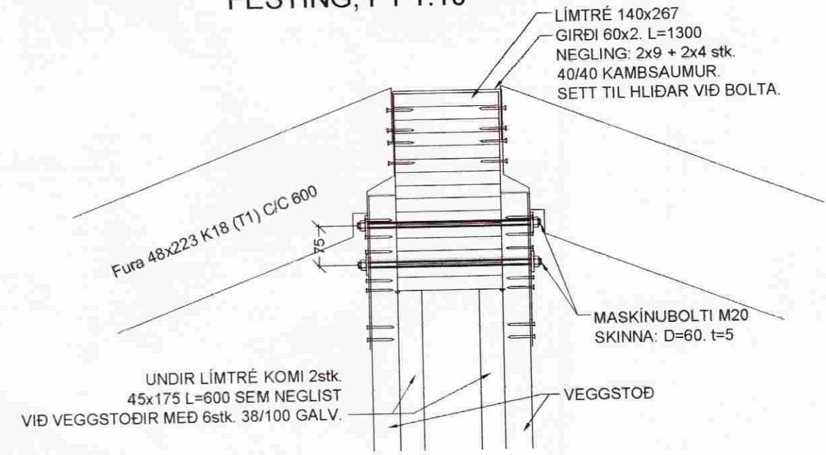
FESTING, F1 1:10
