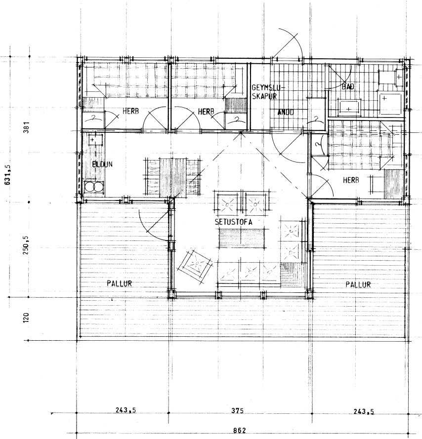
GRUNNMYND M 1:50
