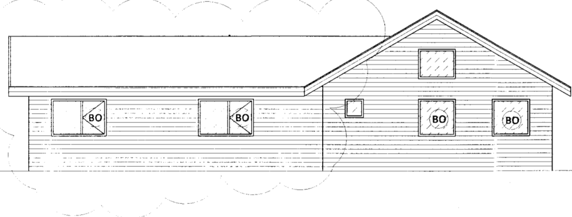
Útlit norðaustur 1:100
