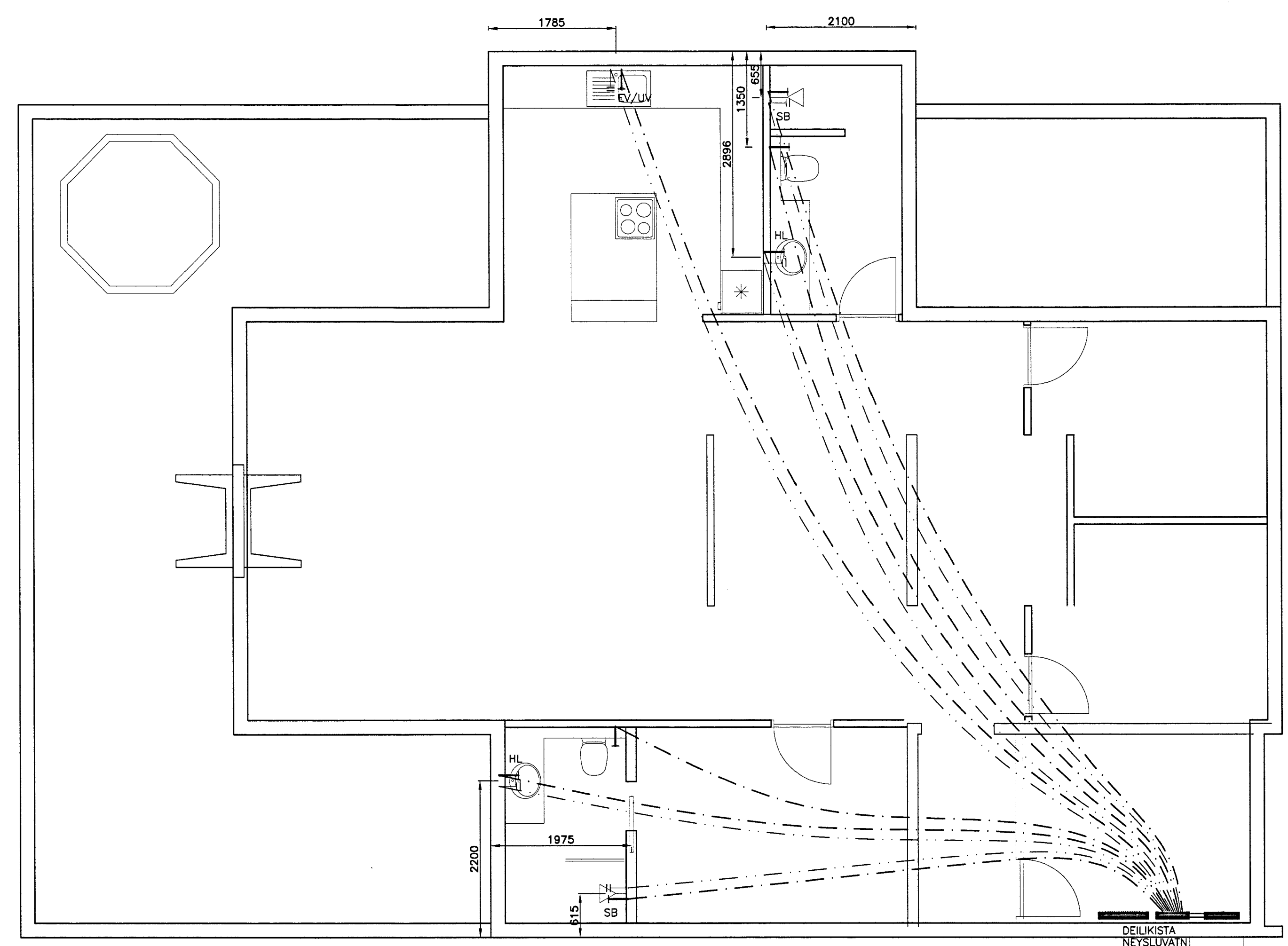
GRUNNMYND NEYSLUVATNSLAGNA MKV. 1:50
