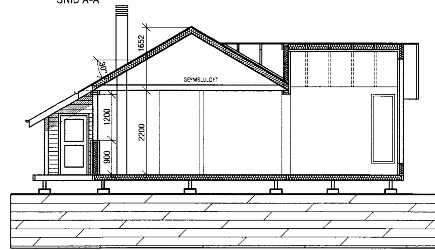
PVERSNID B-B
