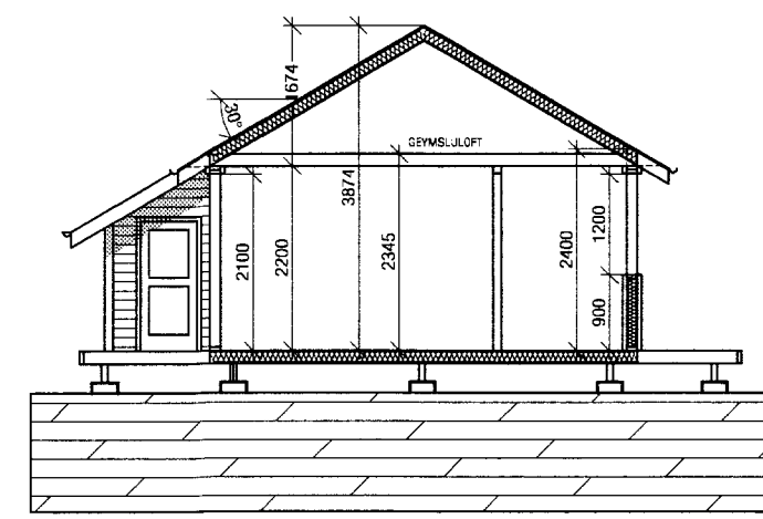
SNID A-A
