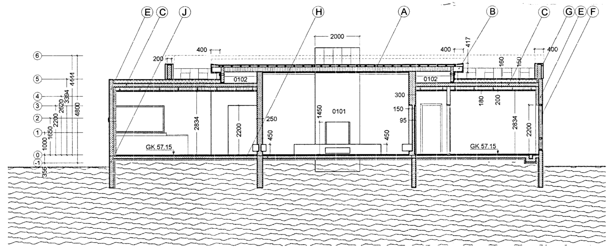
Sneiðmynd B-B
