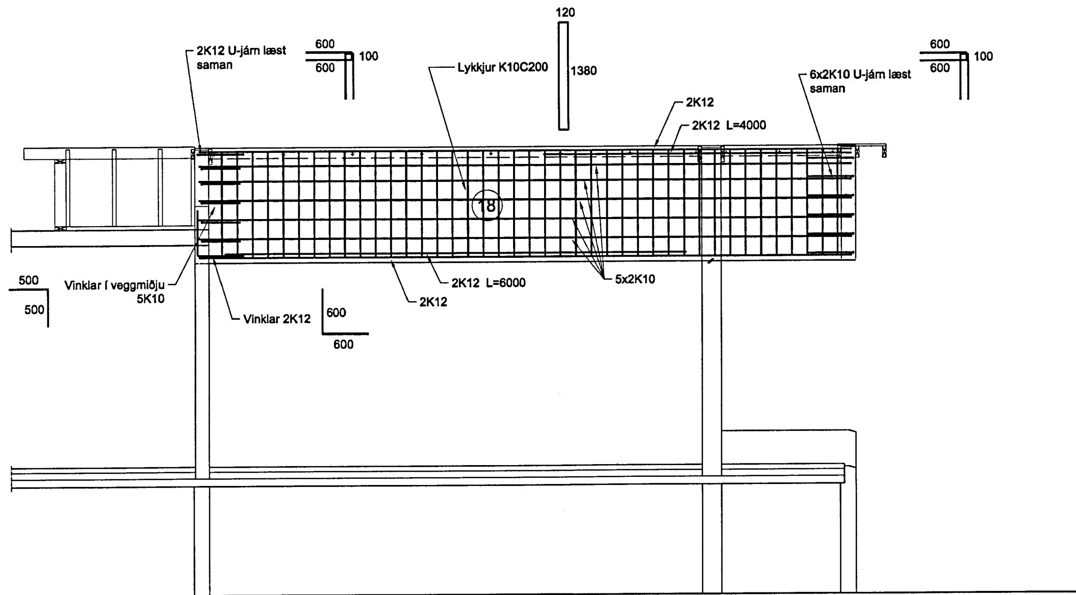
7 LANGSNIÐ 03 Mkv. 1/50
