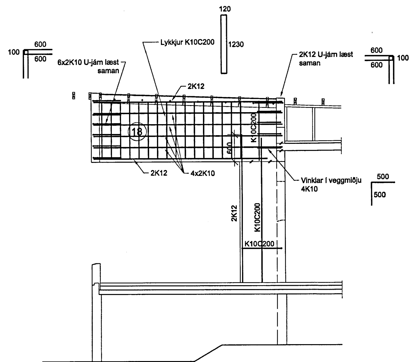
8 LANGSNIÐ 03 Mkv. 1/50
