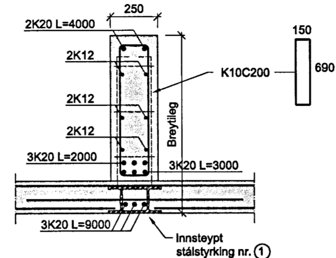
L SNEIÐING 03/04 Mkv. 1/20
