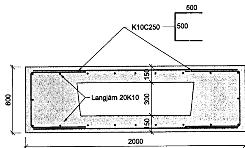
S3 SNEIÐING Í SÚLU 03 Mkv. 1/20
