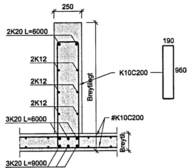
K SNEIÐING 03/04 Mkv. 1/20
