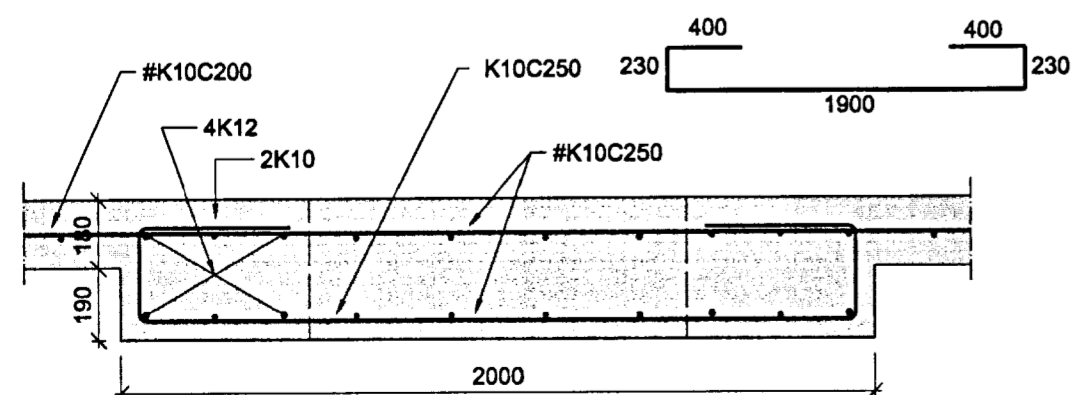
S2 SNEIÐING Í SÚLU 03 Mkv. 1/20
