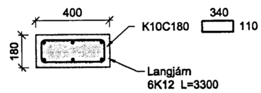
S1 SNEIÐING Í SÚLU 03/05 Mkv. 1/20
