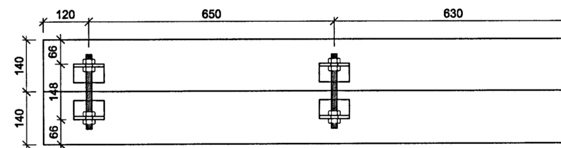
1 SÉRMYND 03 Stálstyrking Mkv. 1/20
