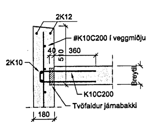
I SNEIÐING 03/04 Mkv. 1/20
