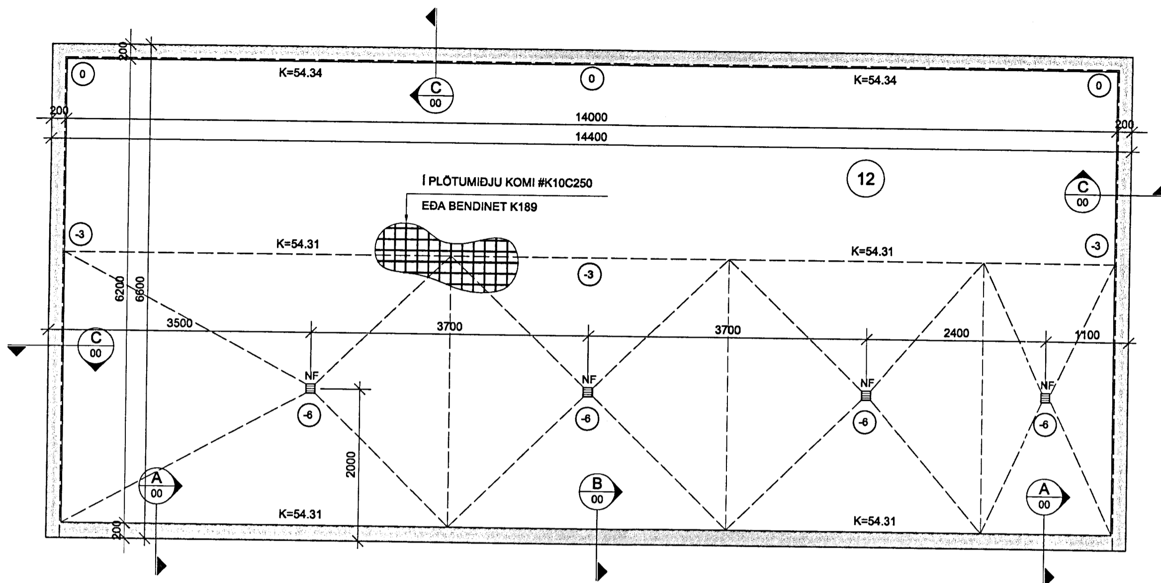
UNDIRSTÖÐUR GRUNNMYND 1:50
