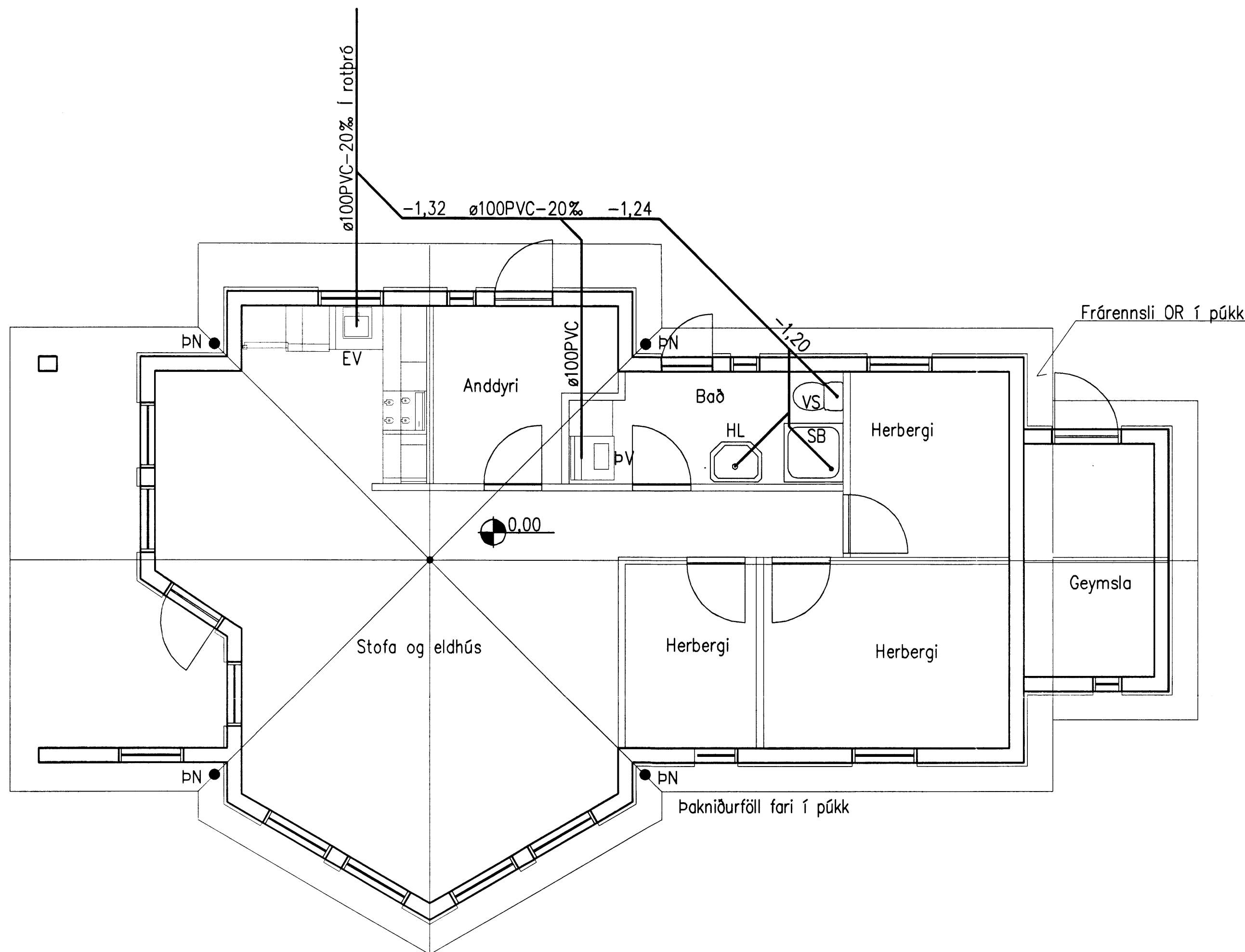
GRUNNMYND – FRÁRENNISLAGNIR, 1:50
