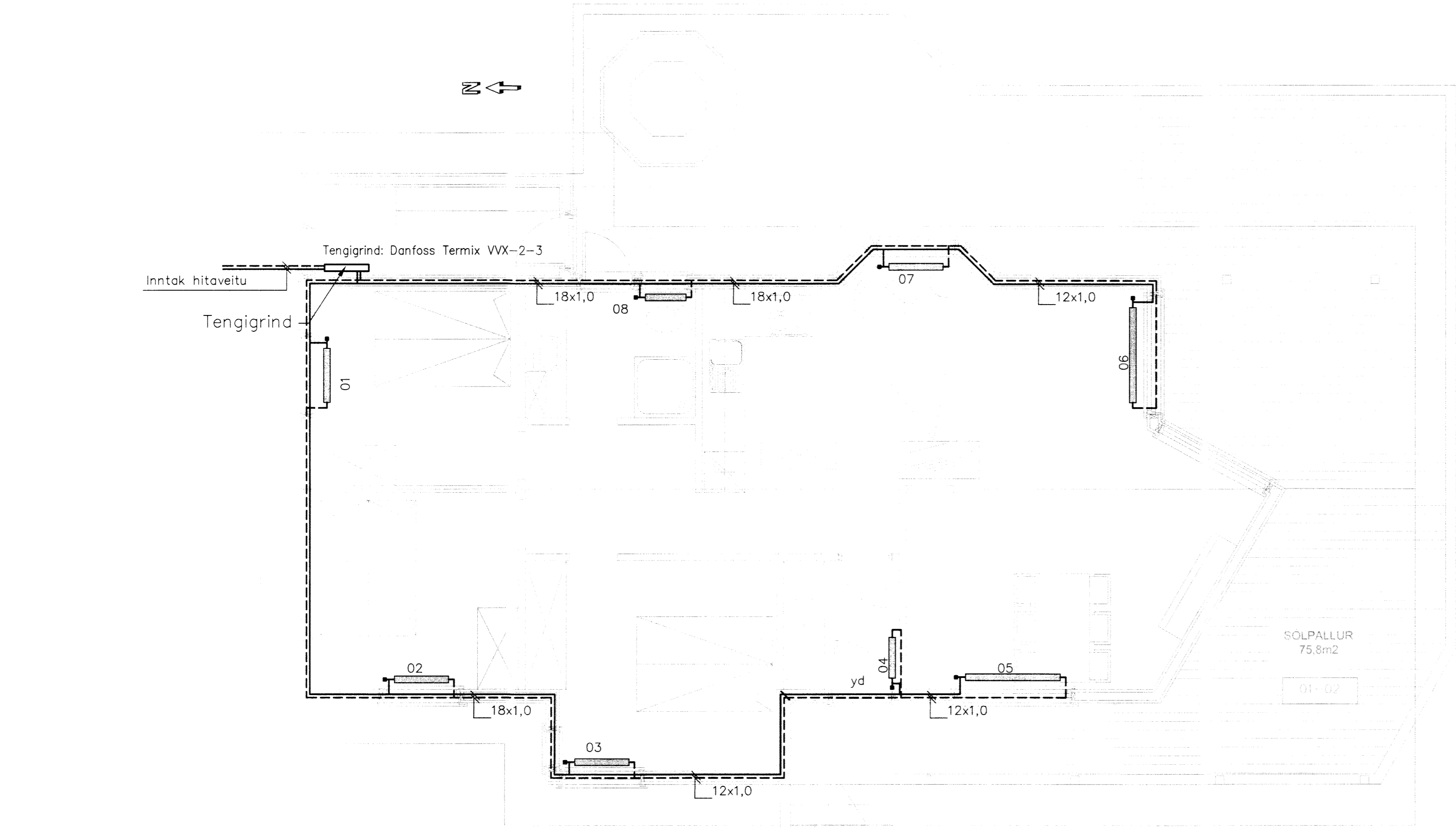
GRUNNMYND OFNLAGNA 1:50
