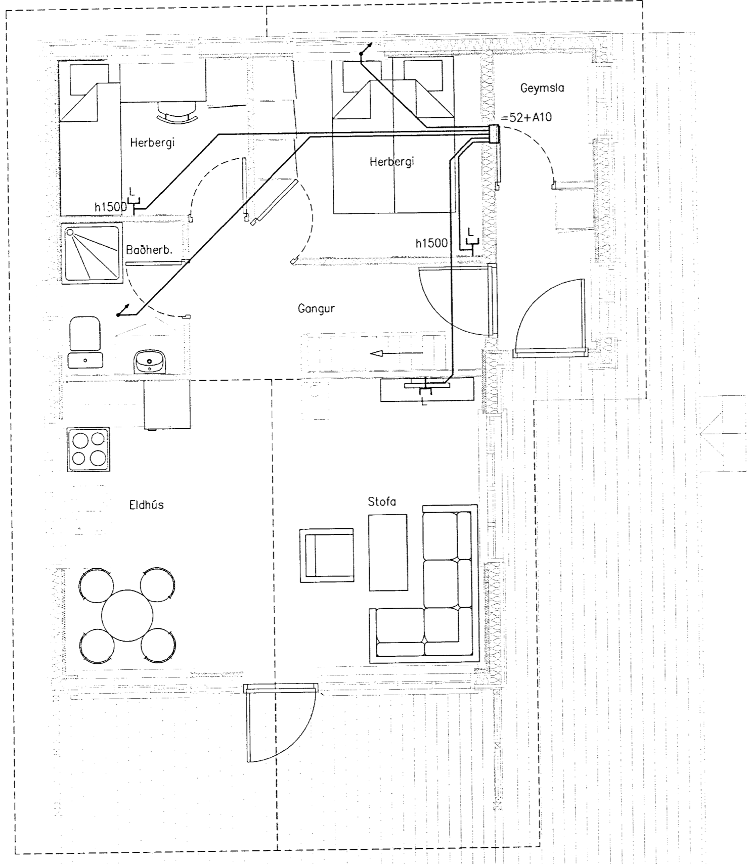
Grunnmynd
