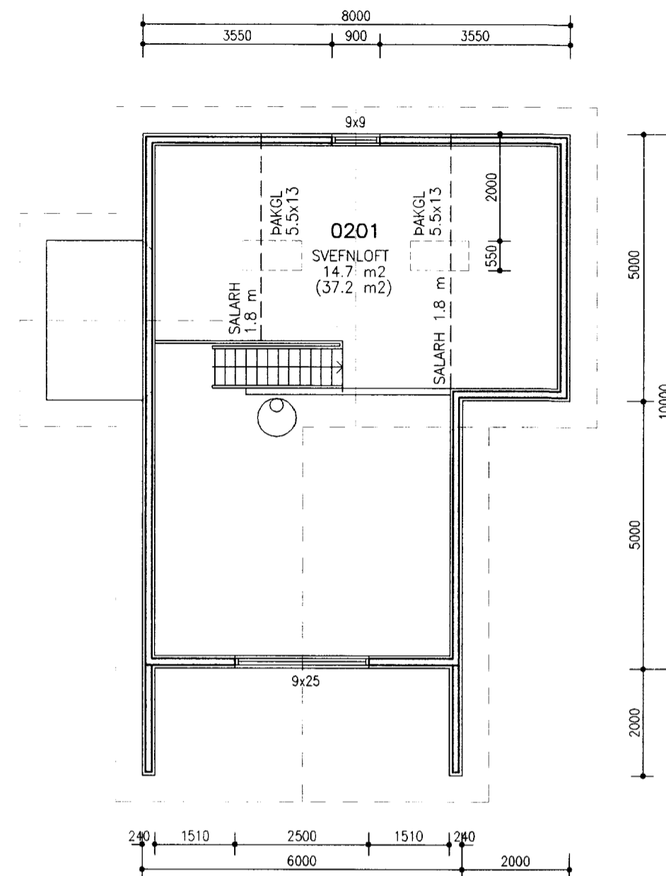
GRUNNMYND 2. HÆÐ 1:100
