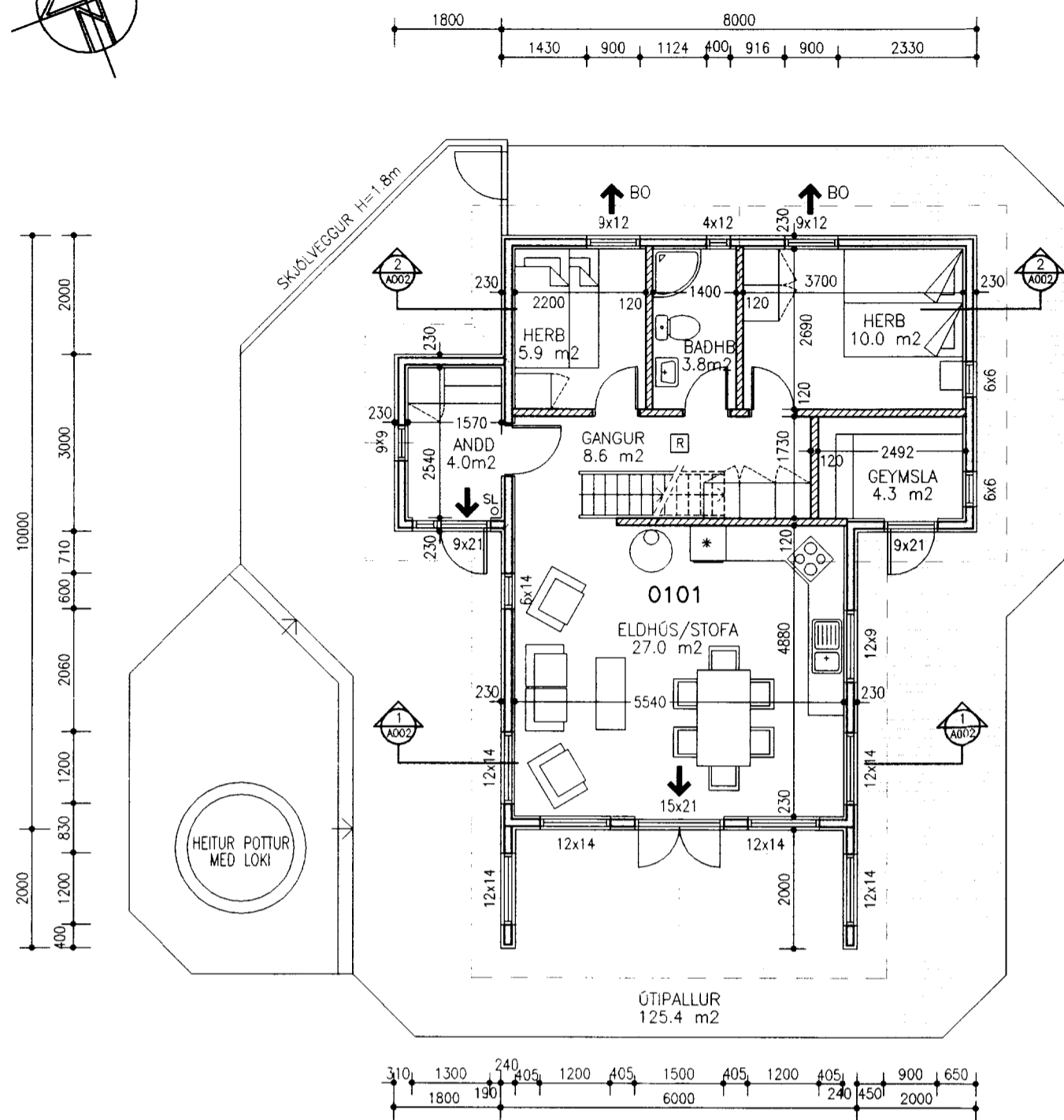
GRUNNMYND 1. HÆÐ 1:100
