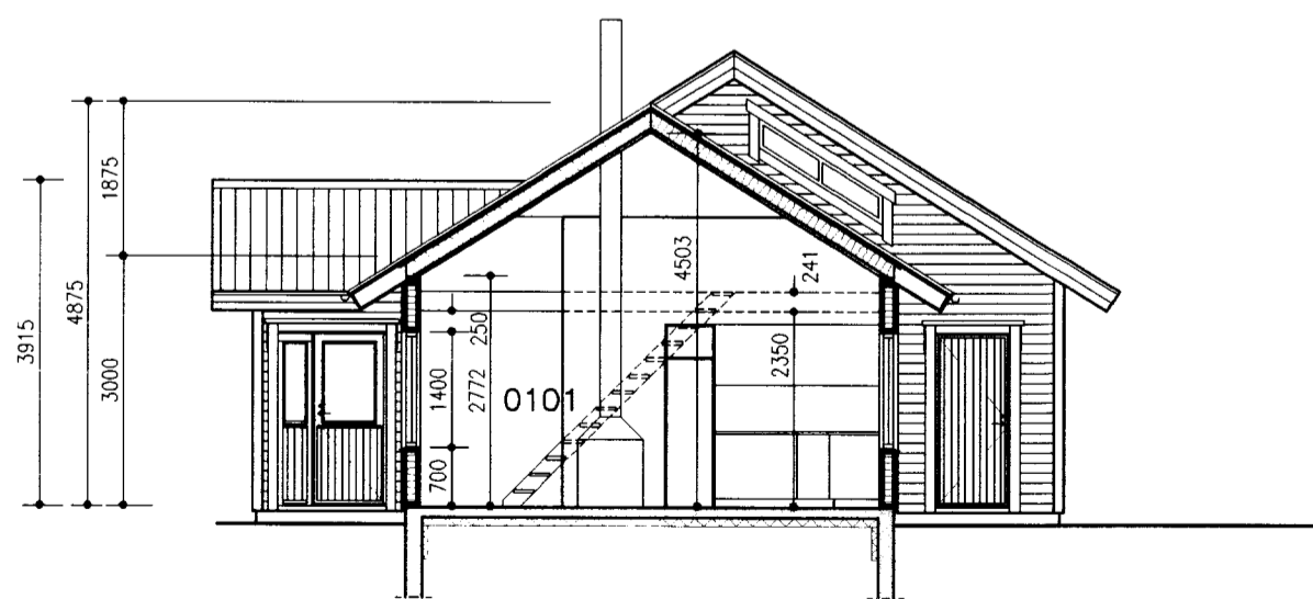
SNID 1-1 1:100
