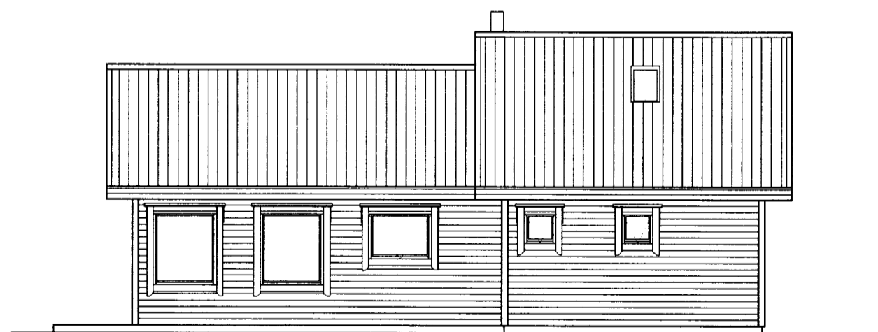
ÚTLIT SUÐAUSTURHLID
