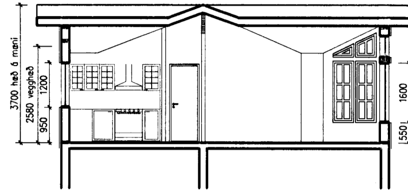
Snið B-B
