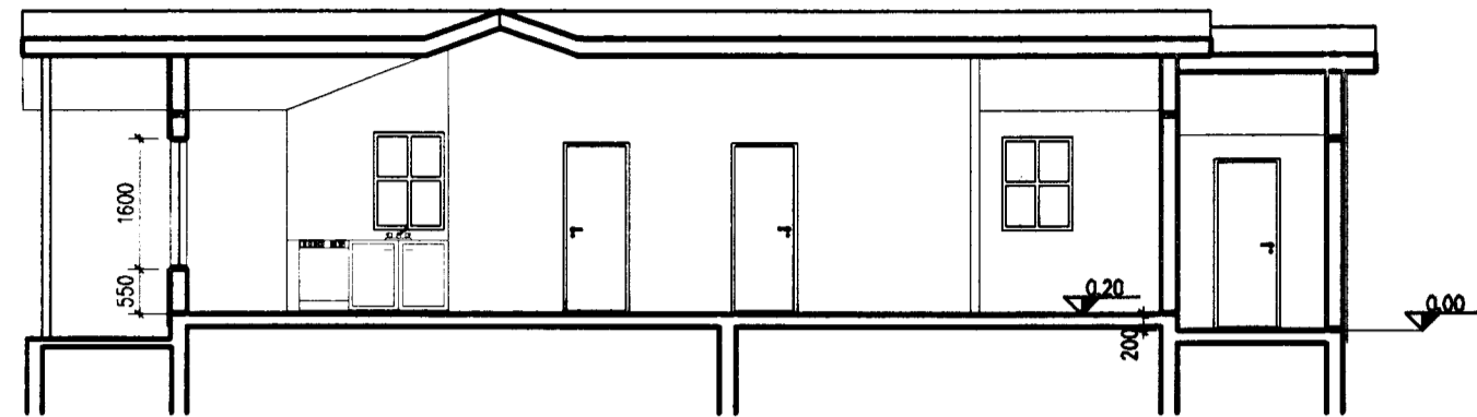
Snið A-A
