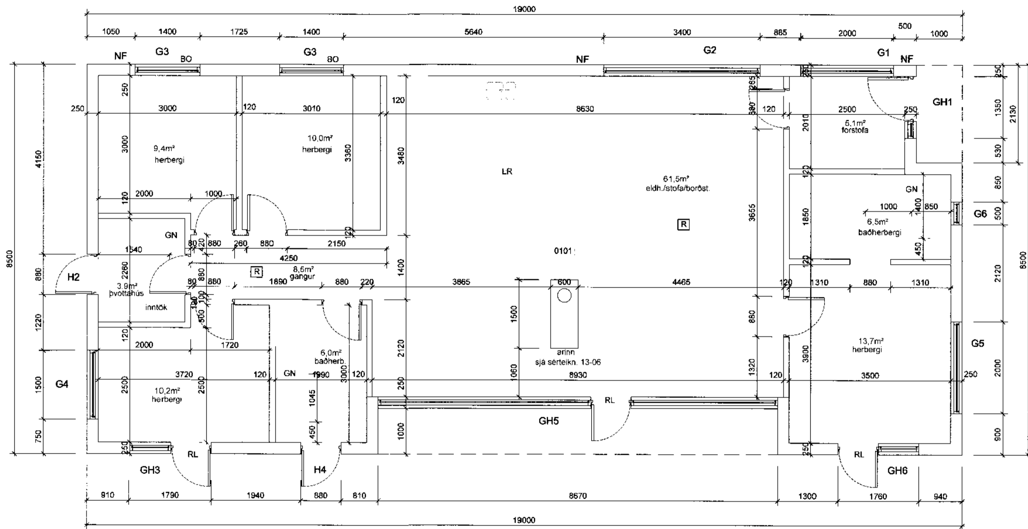
GRUNNMYND 1:50
