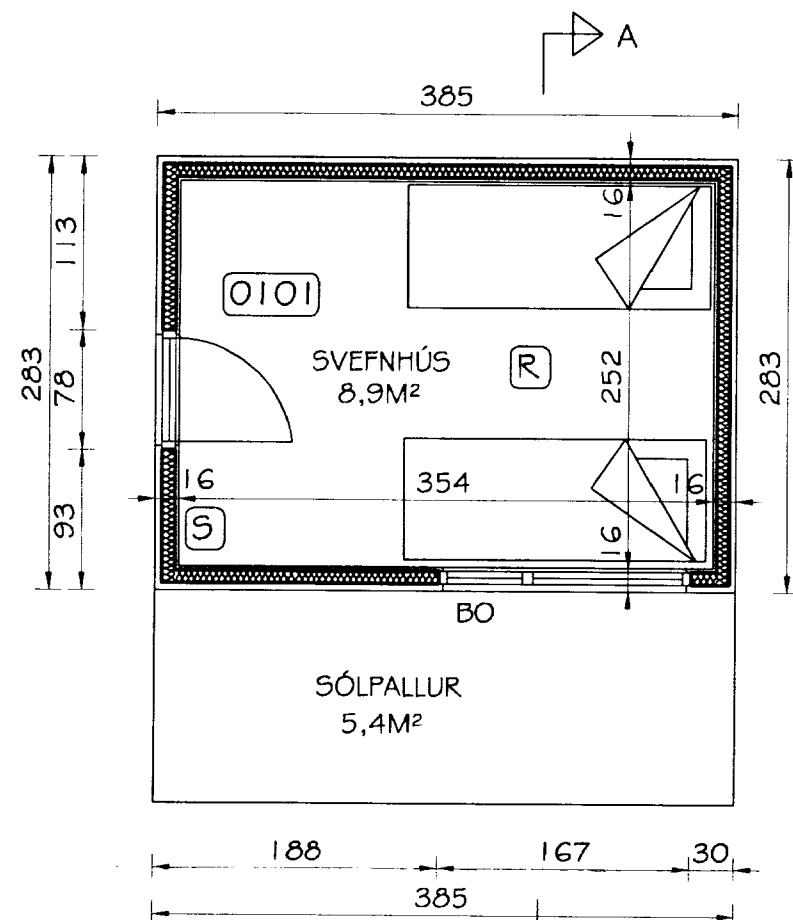
GRUNNMYND MKV. 1:50
