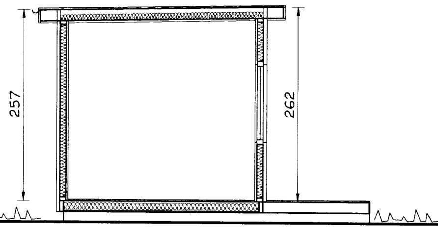
SNID A-A
