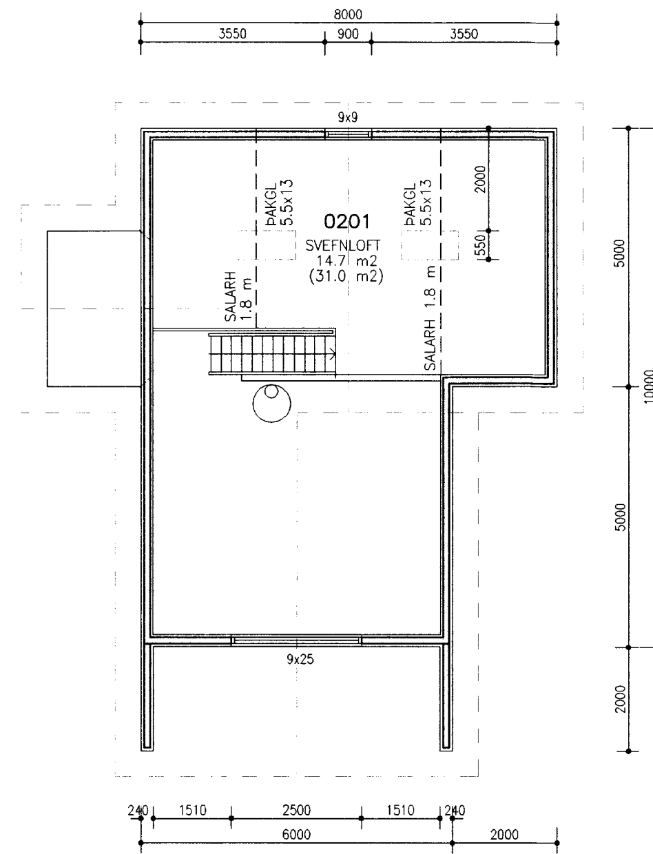
GRUNNMYND 2. HÆÐ 1:100
