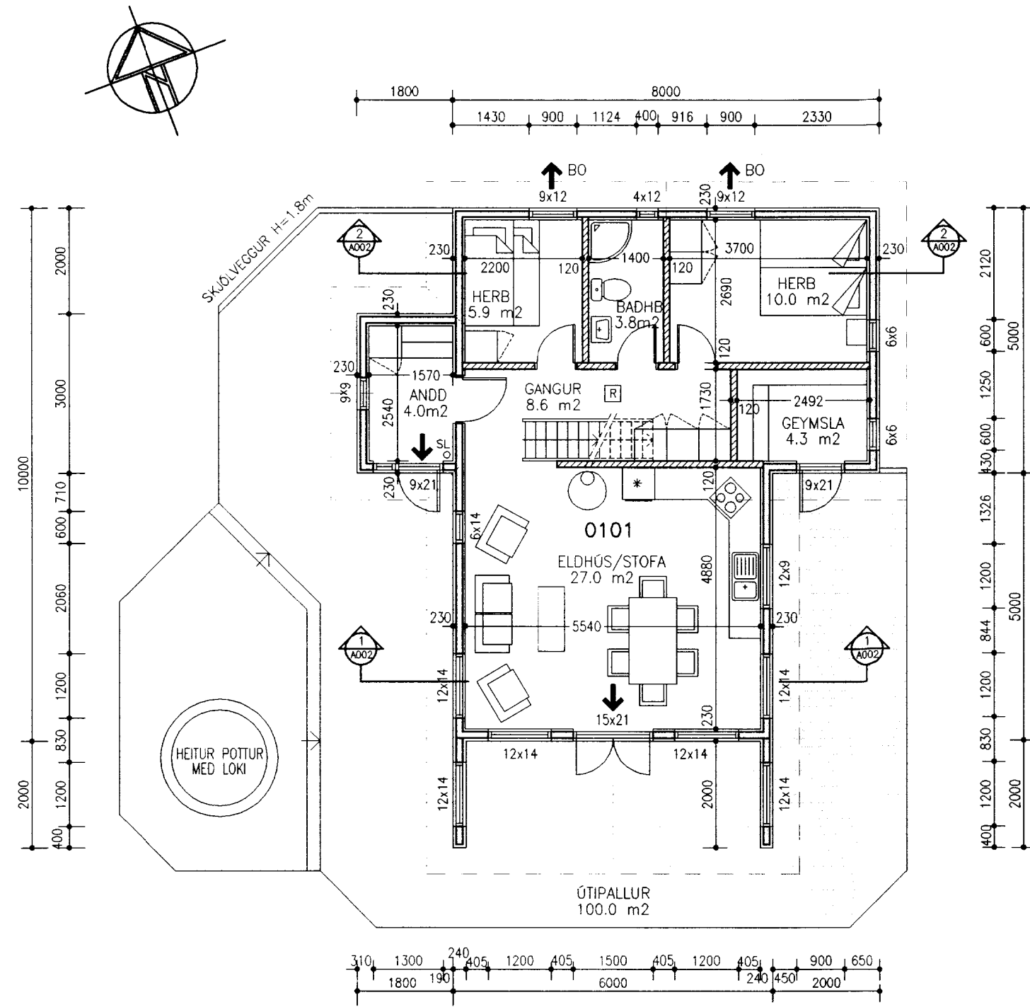
GRUNNMYND 1. HÆÐ 1:100
