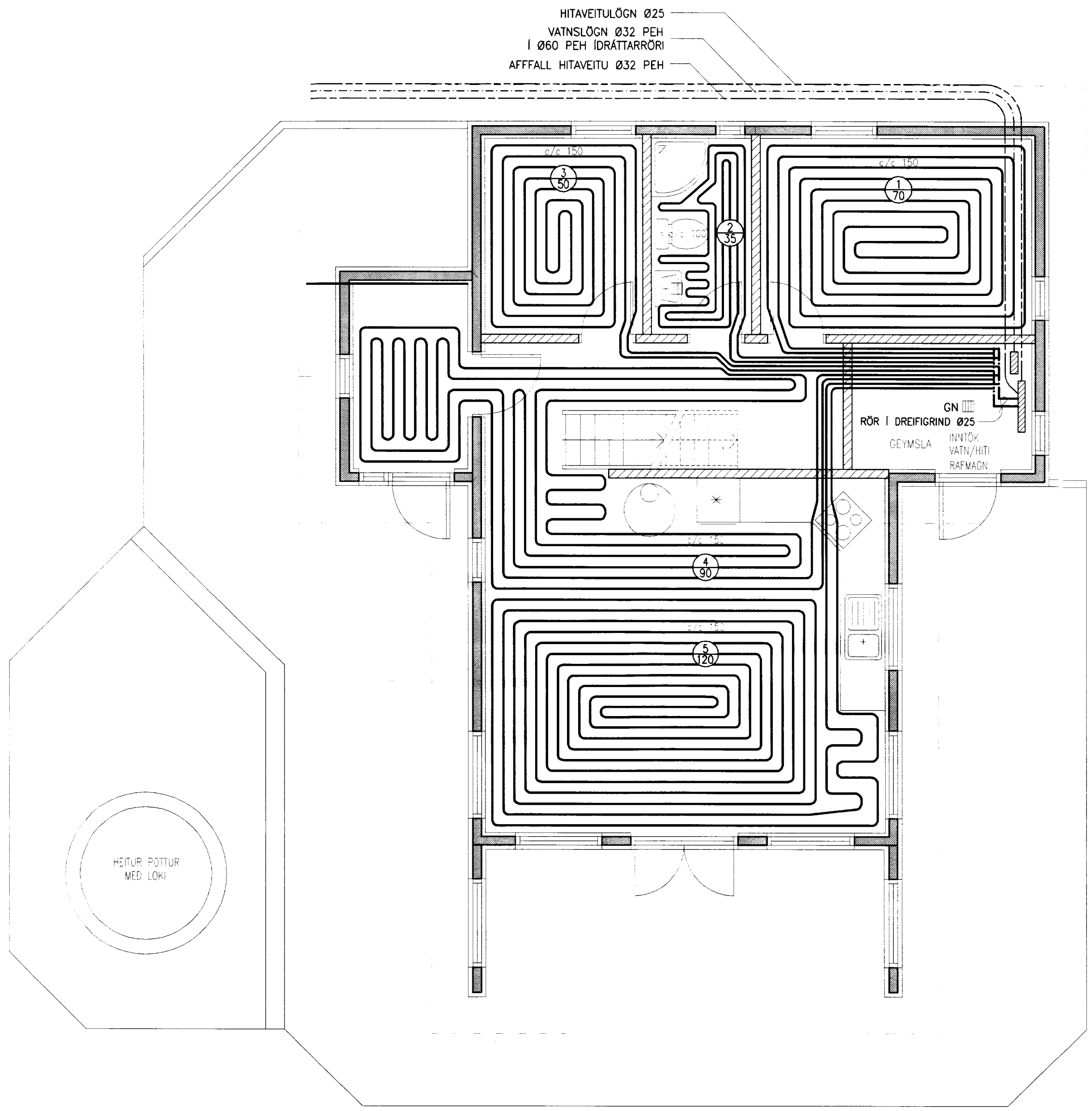
GRUNNMYND VATNSLAGNIR 1:50
