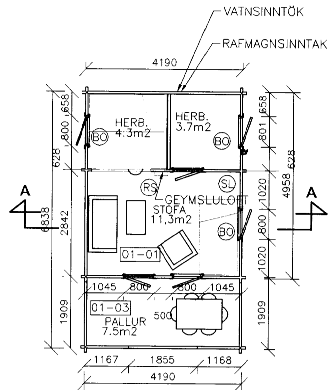
GRUNNMYND 1:100
