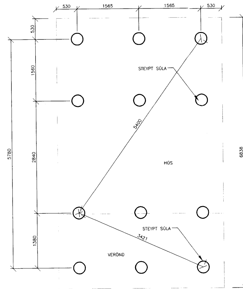
GRUNNMYND STEYPTAR SÚLUR 1:50
