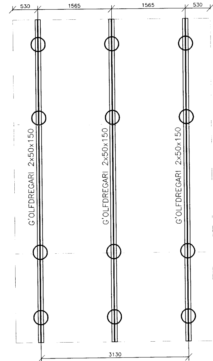
GRUNNMYND DREGARAR 1:50
