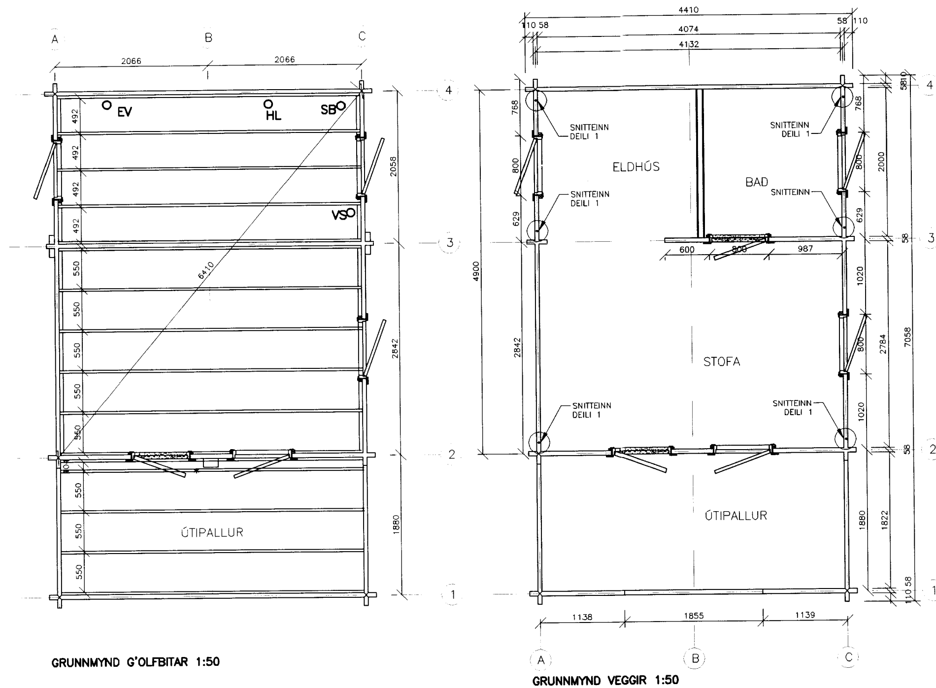
GRUNNMYND VEGGIR 1:50
