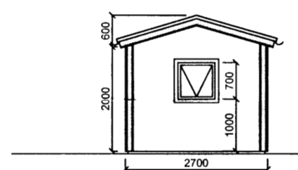
SNID A-A
