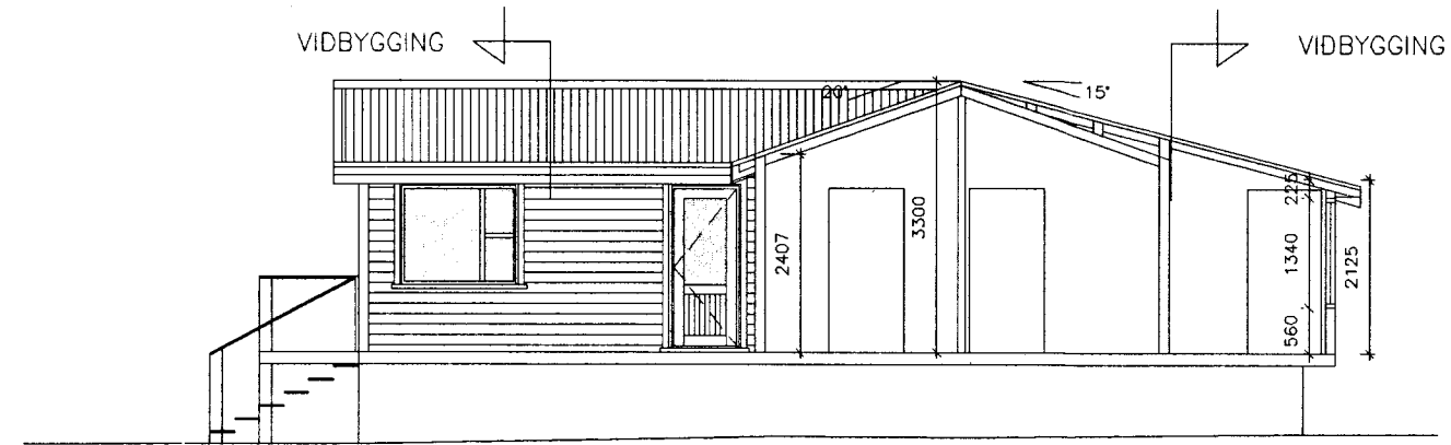
SNID A-A Mkv 1:100
