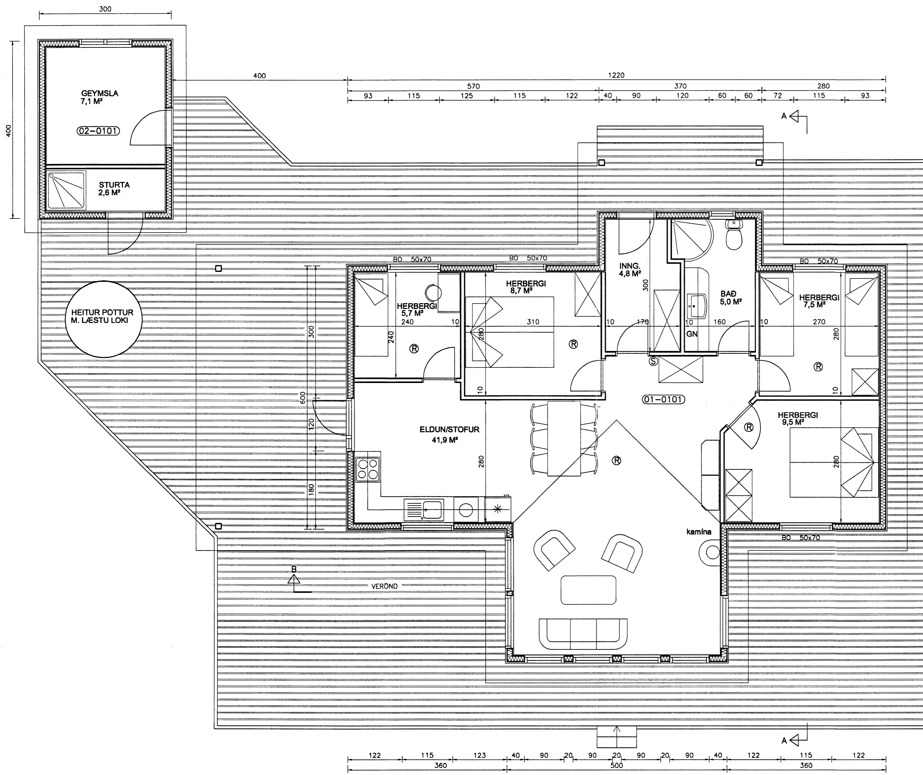
GRUNNMYND mkv. 1:100
