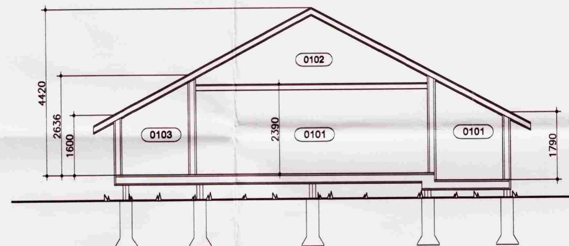
SNEIÐING A-A
