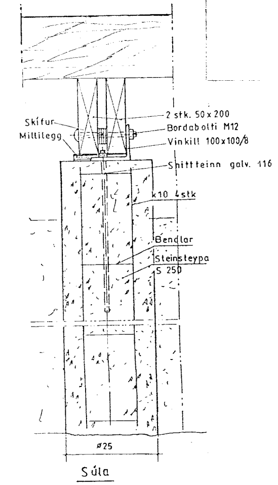
Snid A-A
