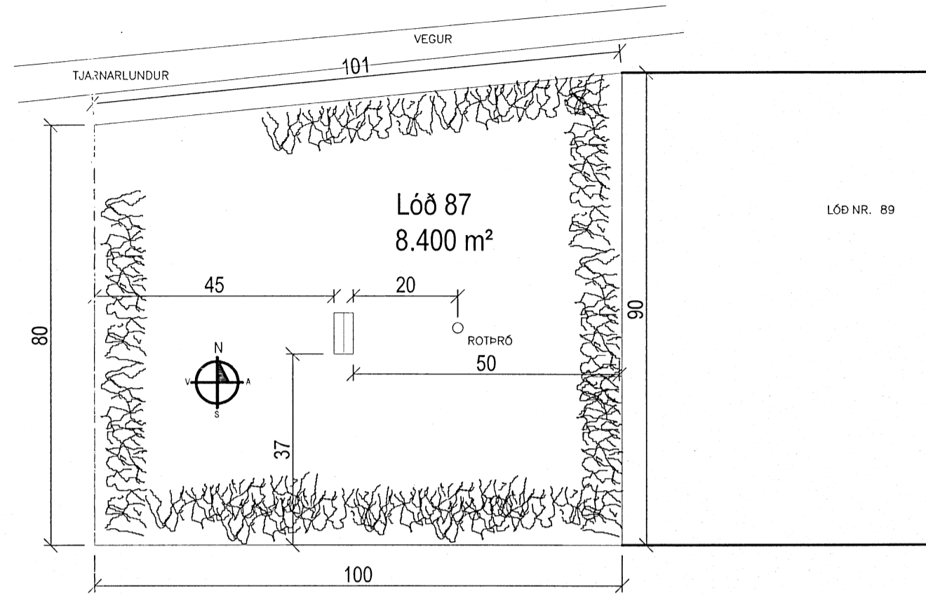
Afstöðumynd, lóð 87 M= 1:1000
