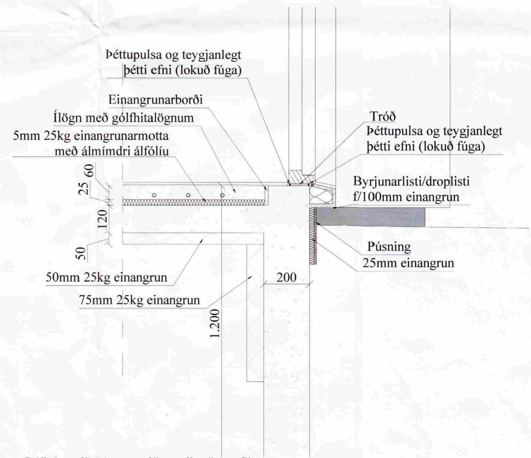
Lóðrétt snið í útvegg við rennihurð á gaffli.
