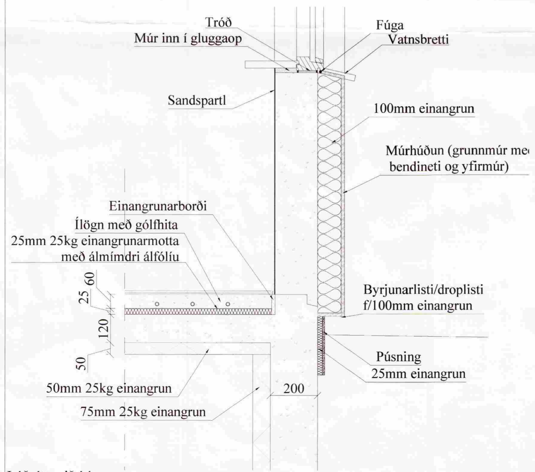
Lóðrétt snið í útvegg.
