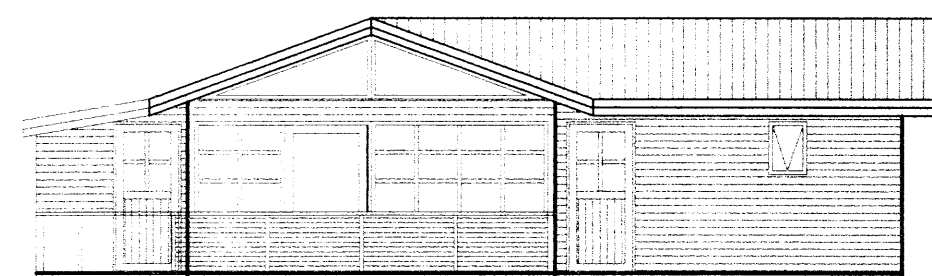
Útlit suðurhlíð mkv. 1:100
