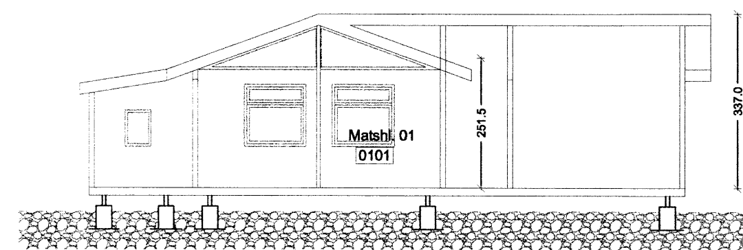
Sneiðing A - A mkv. 1:100
