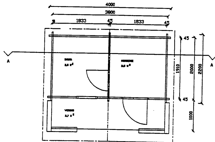
Grunnmynd
