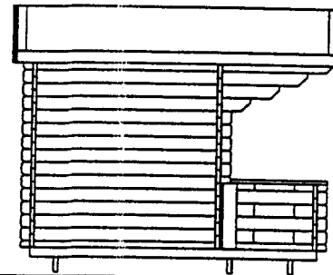
Hliðarmynd
