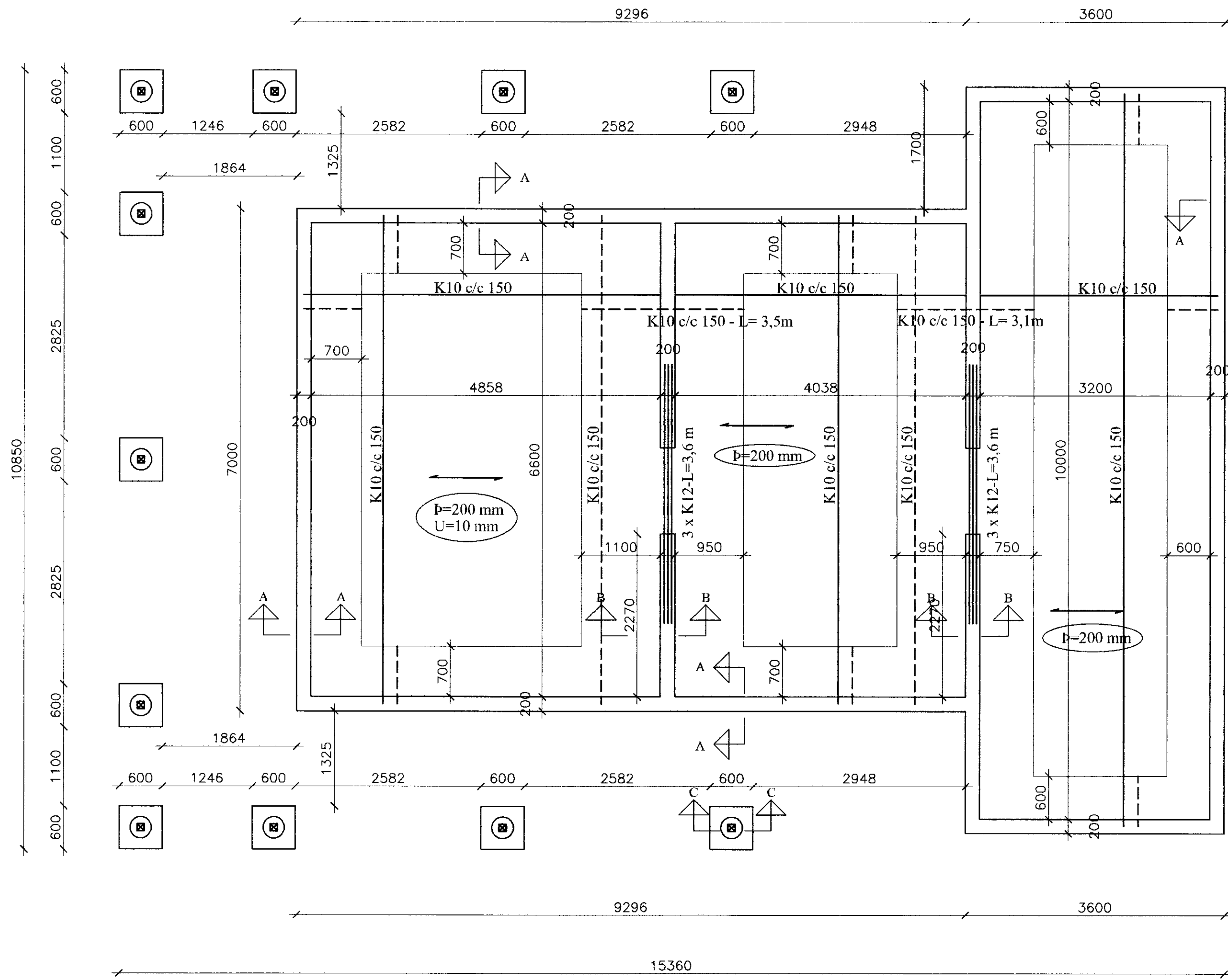
GRUNNMYND SÖKKLA. Mkv. 1:50
