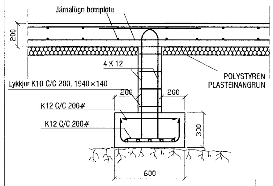
Mkv 1:20 B-B
