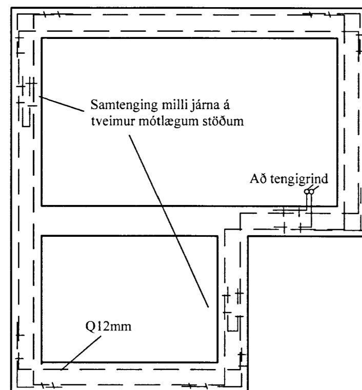
Grunnmynd sökkulveggja
