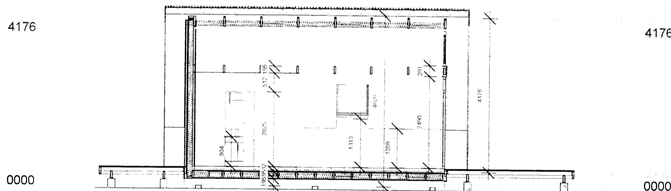
Snið B-B 1 : 100
