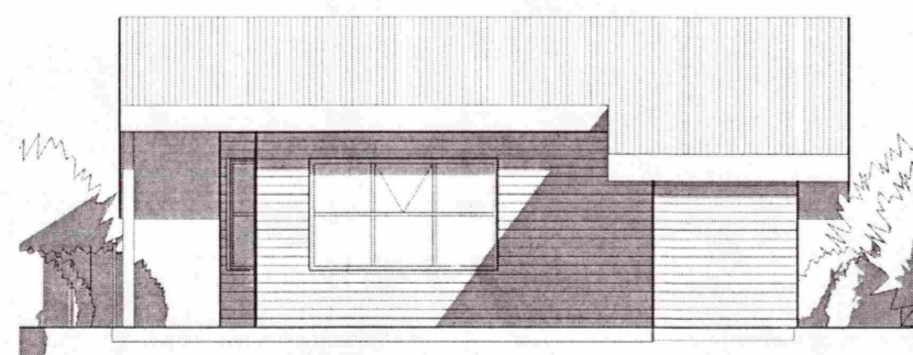
4 Suður 1 : 100
