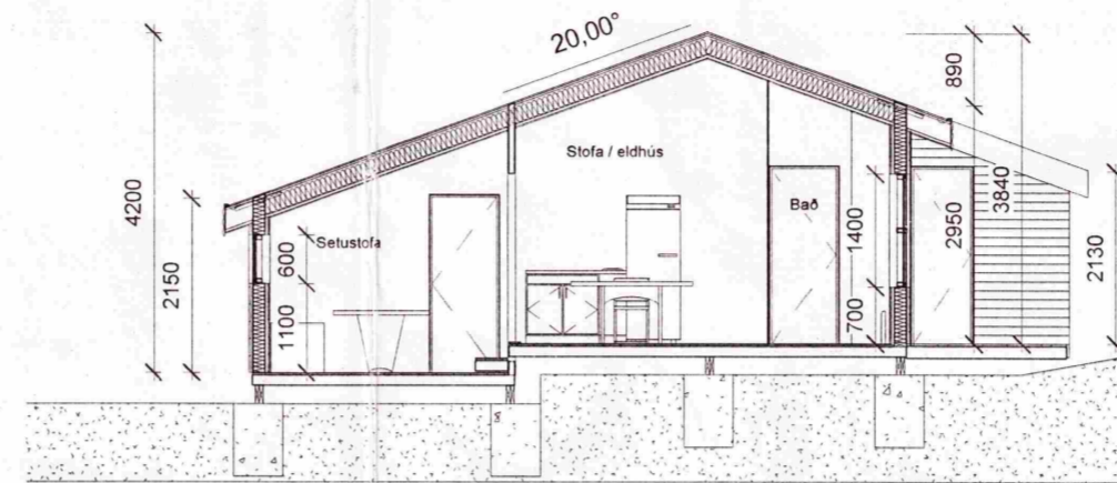
6 Sneiðing 1 : 100
