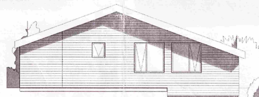
2 Austur 1 : 100
