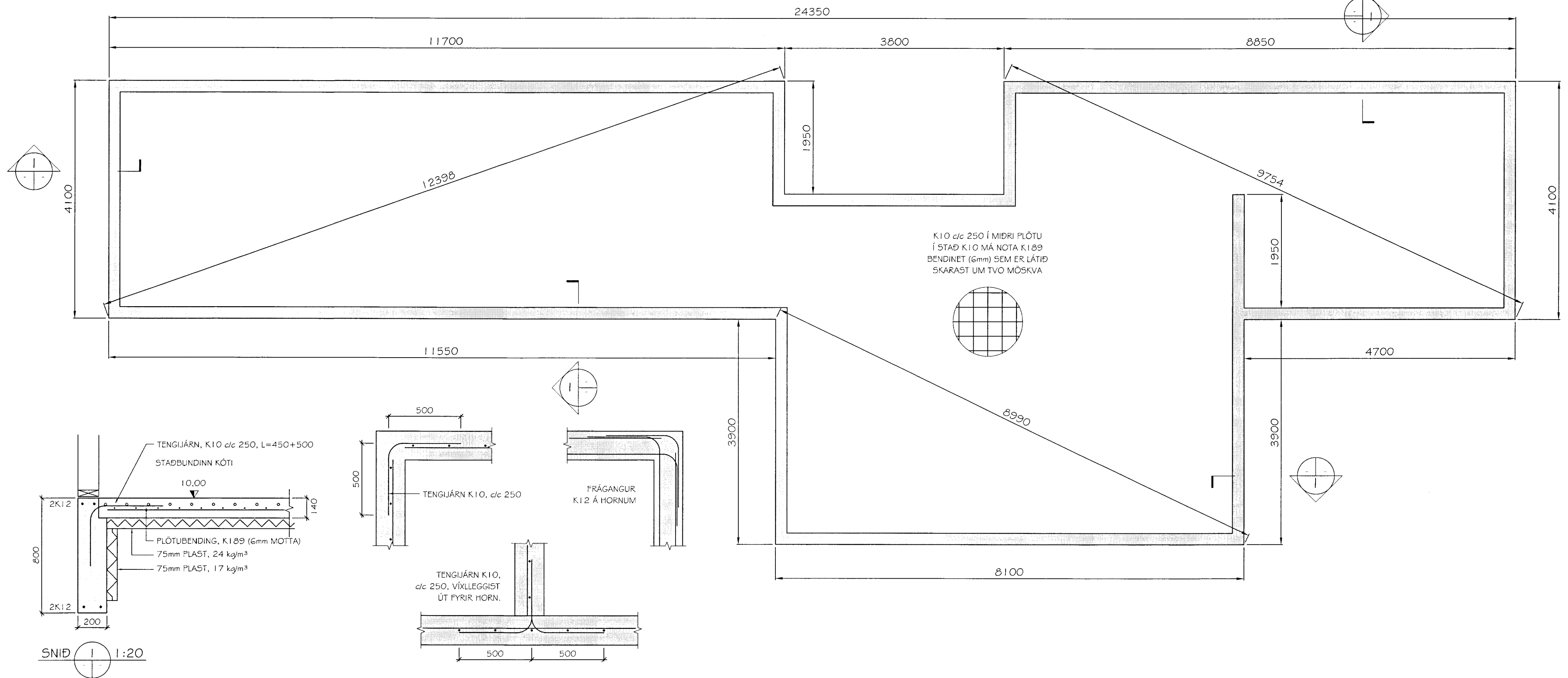
FRÁGANGUR JÁRNA Á HORNUM OG T-TENGLINGU Mkv 1:20
