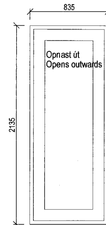
H-02, 2.stk M= 1:25
