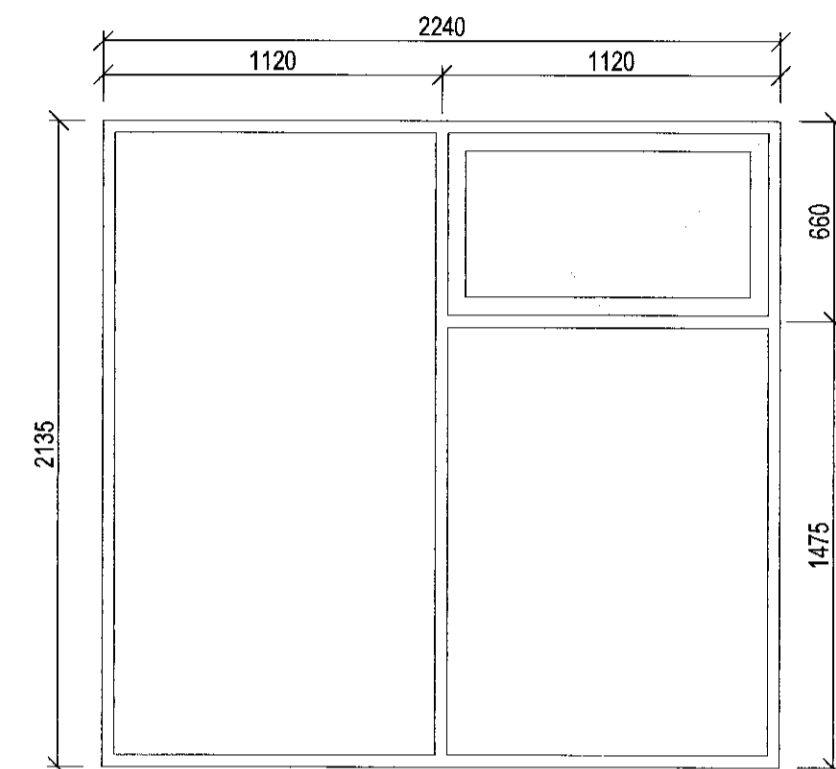
G-05, 2.stk M= 1:25
