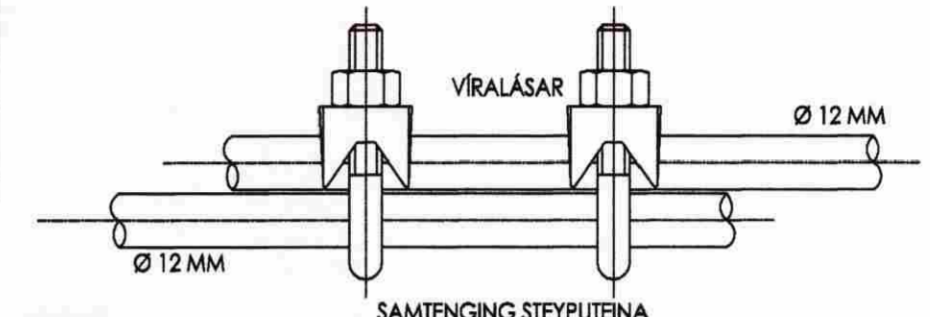
SETJA SKAL TVO VÍRALÁSA Á HVER SAMSKYTTI.
