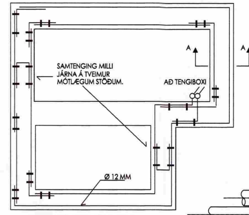
GRUNNMYND SÖKKULVEGGJA
