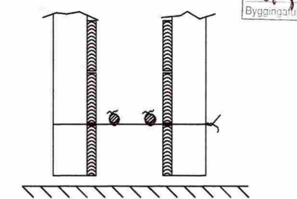
SNID A-A Í SÖKKULVEGG SÝND ERU 2 NEDSTU STEYPUSTYRKARJÁRN Í STEYPUMÓTI OFAN Á NEDSTU MÖTAVÍRUM.
