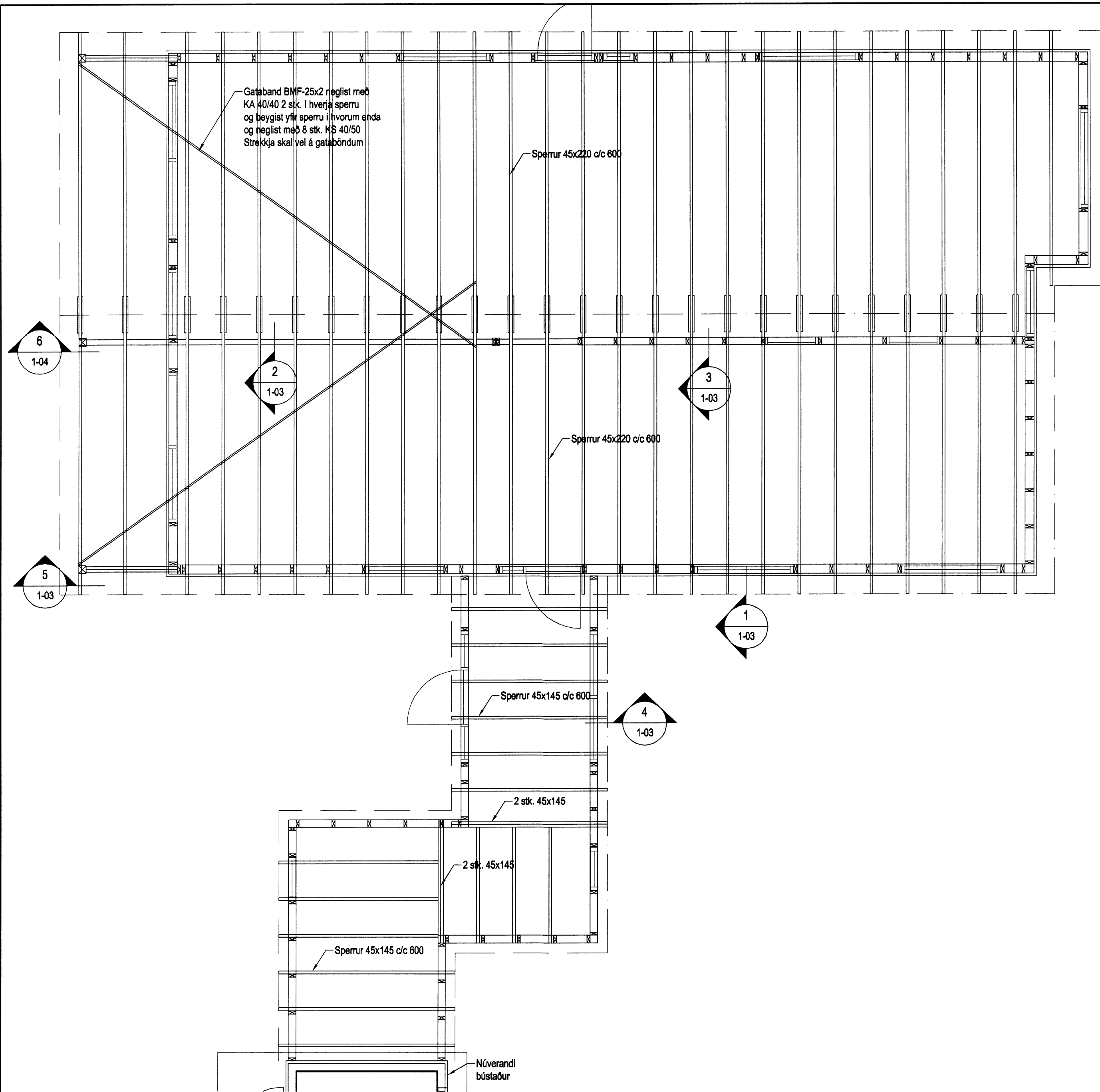
Þakvirki, Grunnmynd, 1:50
