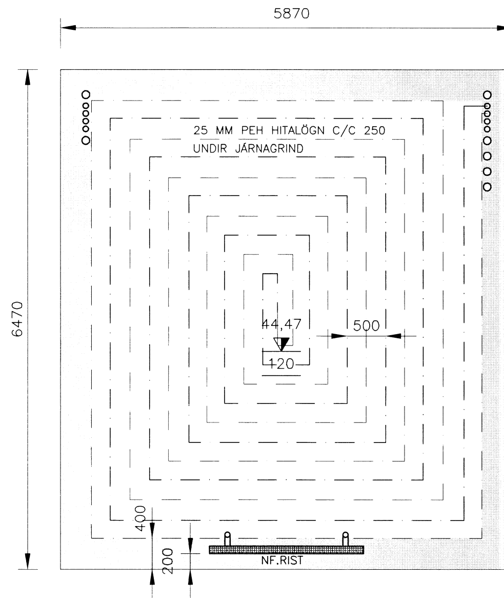
HITALÖGN I GÓLFI GRUNNMYND, 1:50
