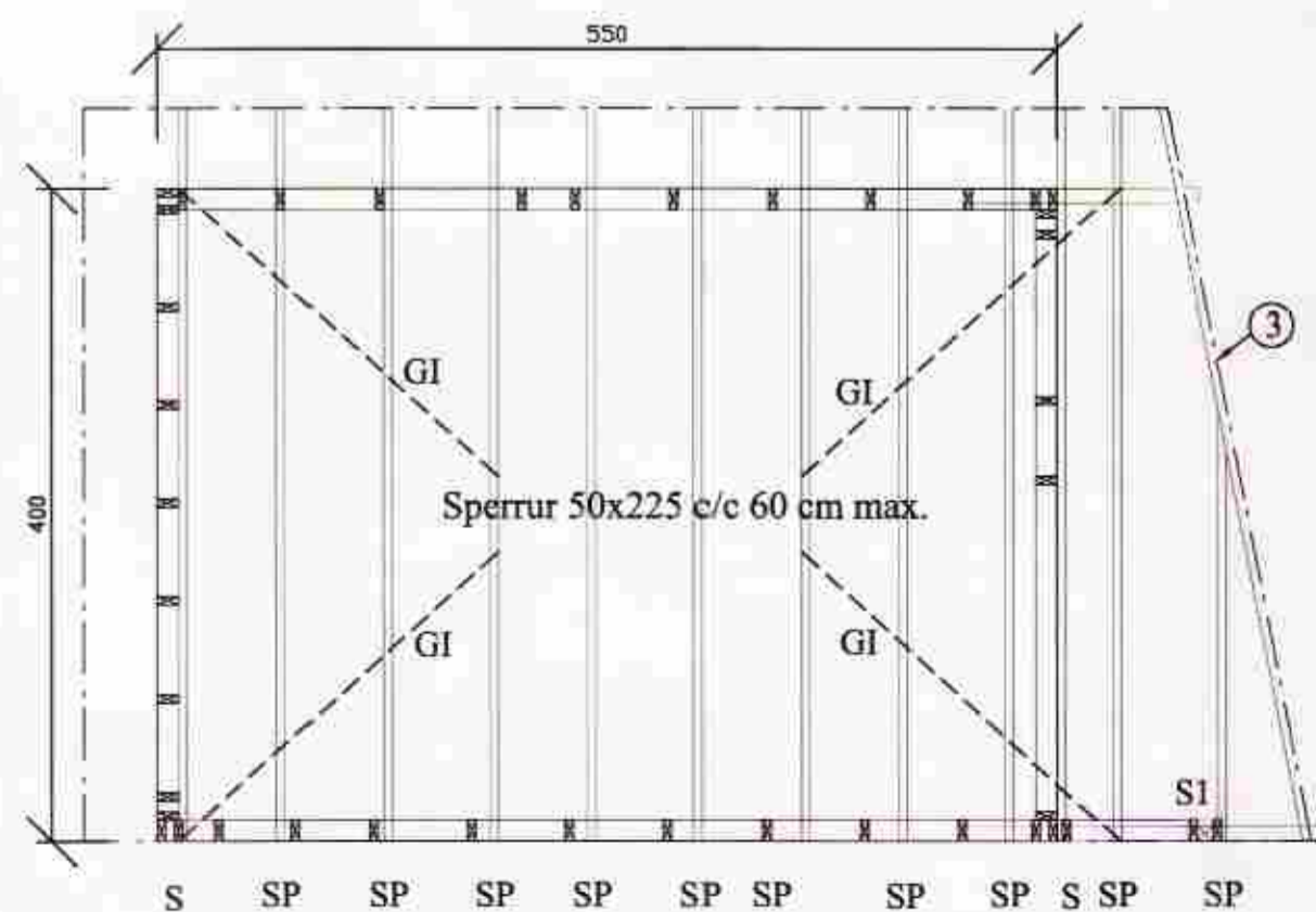
GRUNNMYND ÞAK
