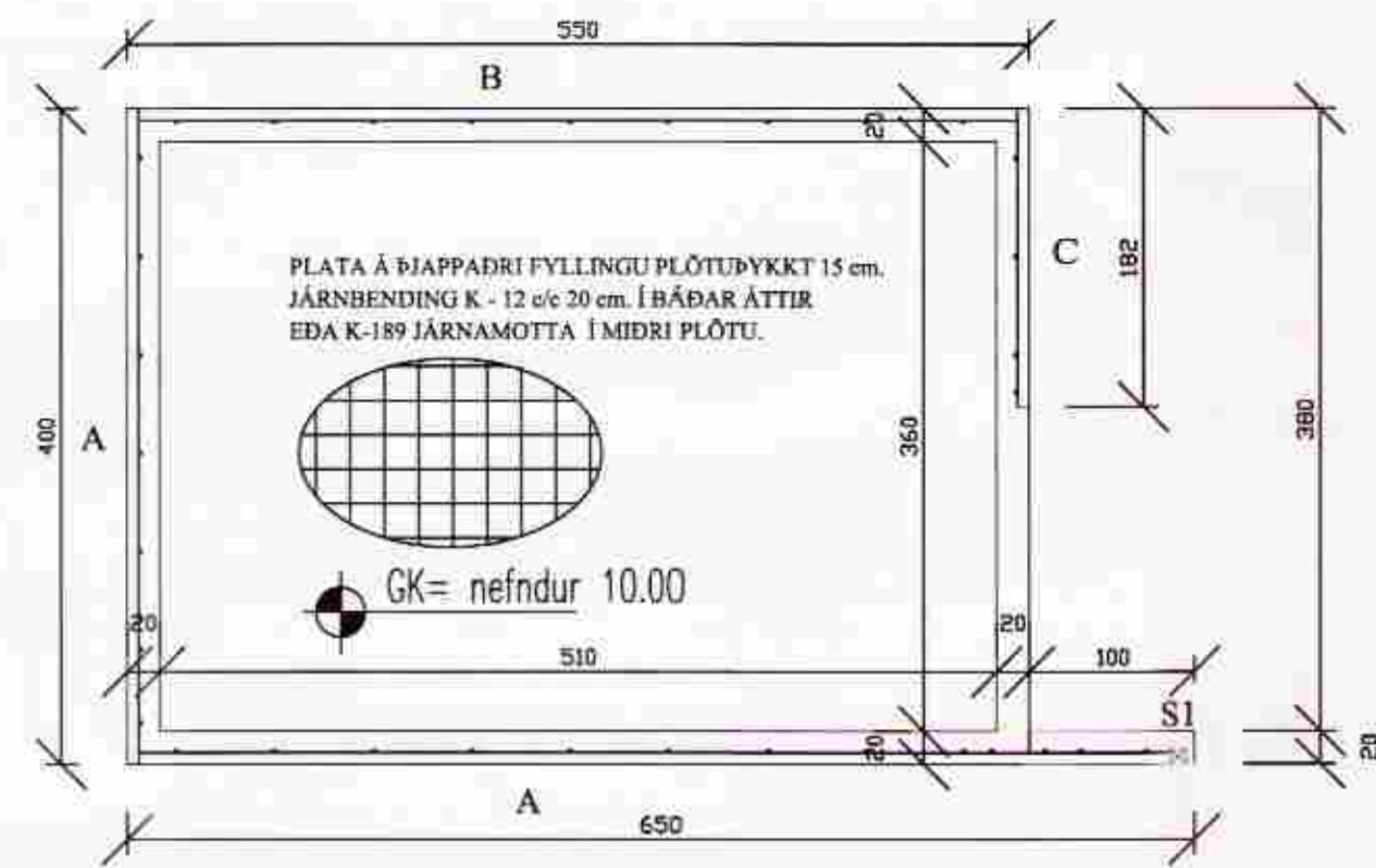
GRUNNMYND SÖKKLAR
