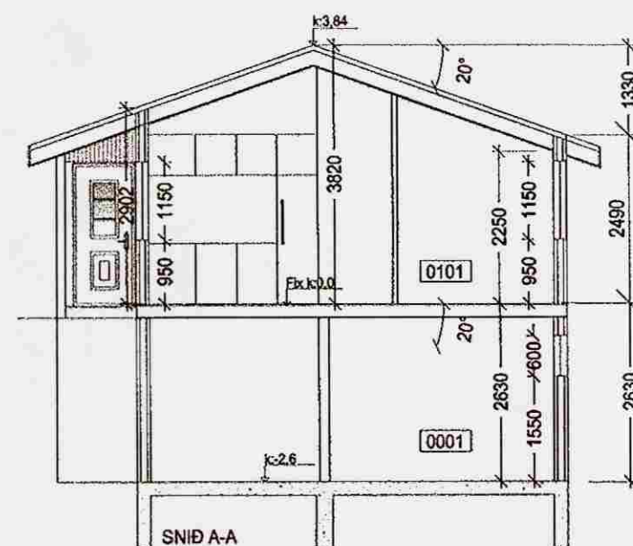
SNID A-A
