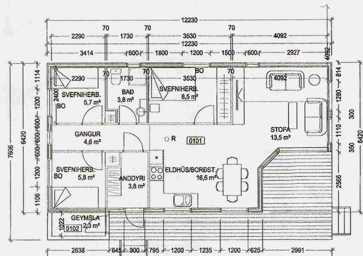
GRUNNMYND 1 HÆÐ
