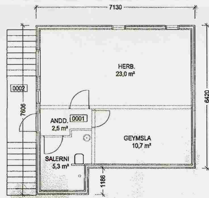
GRUNNMYND KJALLARI
