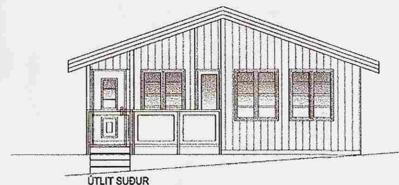
ÚTLIT SUÐUR
