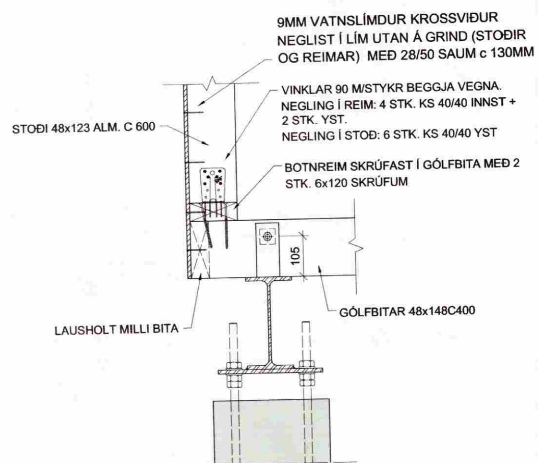
D1 DEILI 00 Mkv. 1/10
