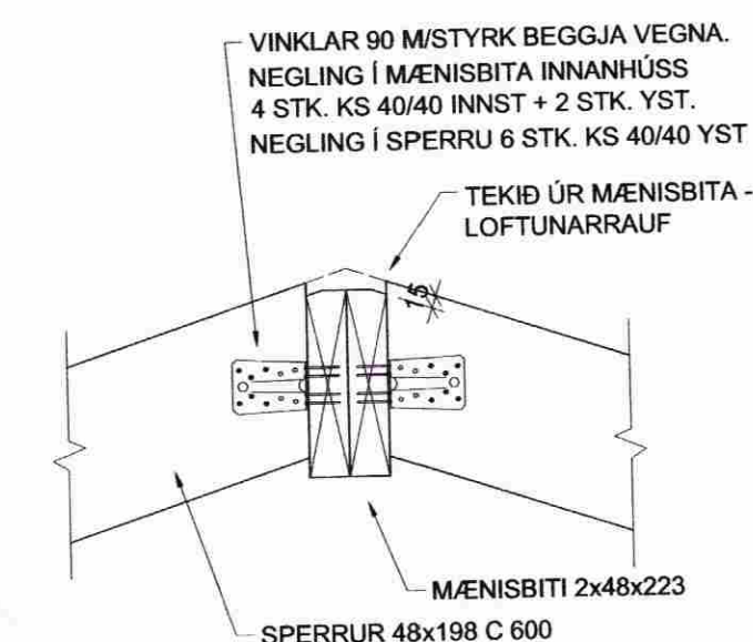
D3 DEILI 00 Mkv. 1/10
