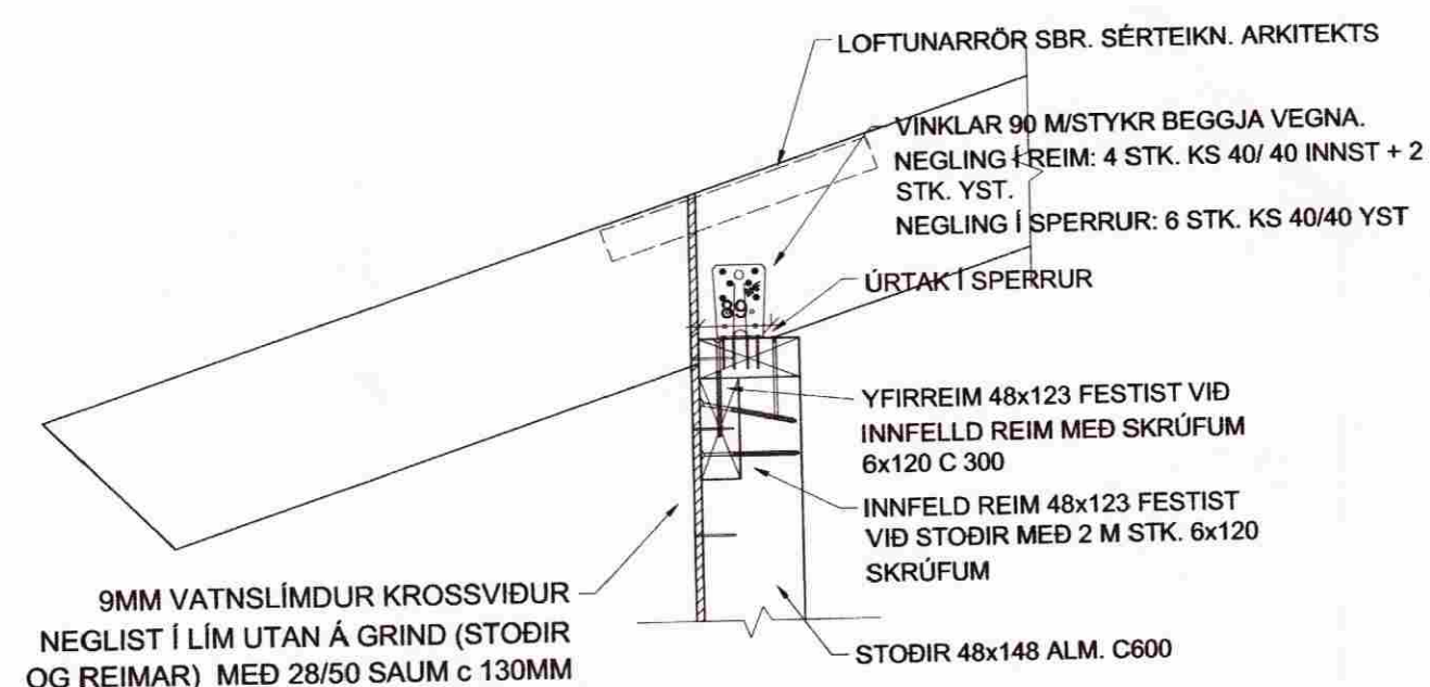
D2 DEILI 00 Mkv. 1/10
