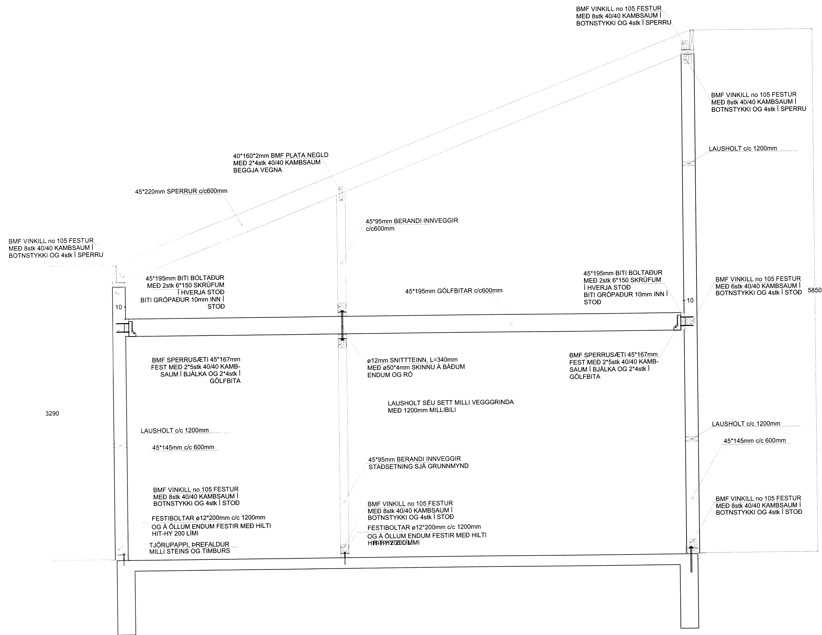
S1 SNEIÐING Í GRIND mkv 1:20
