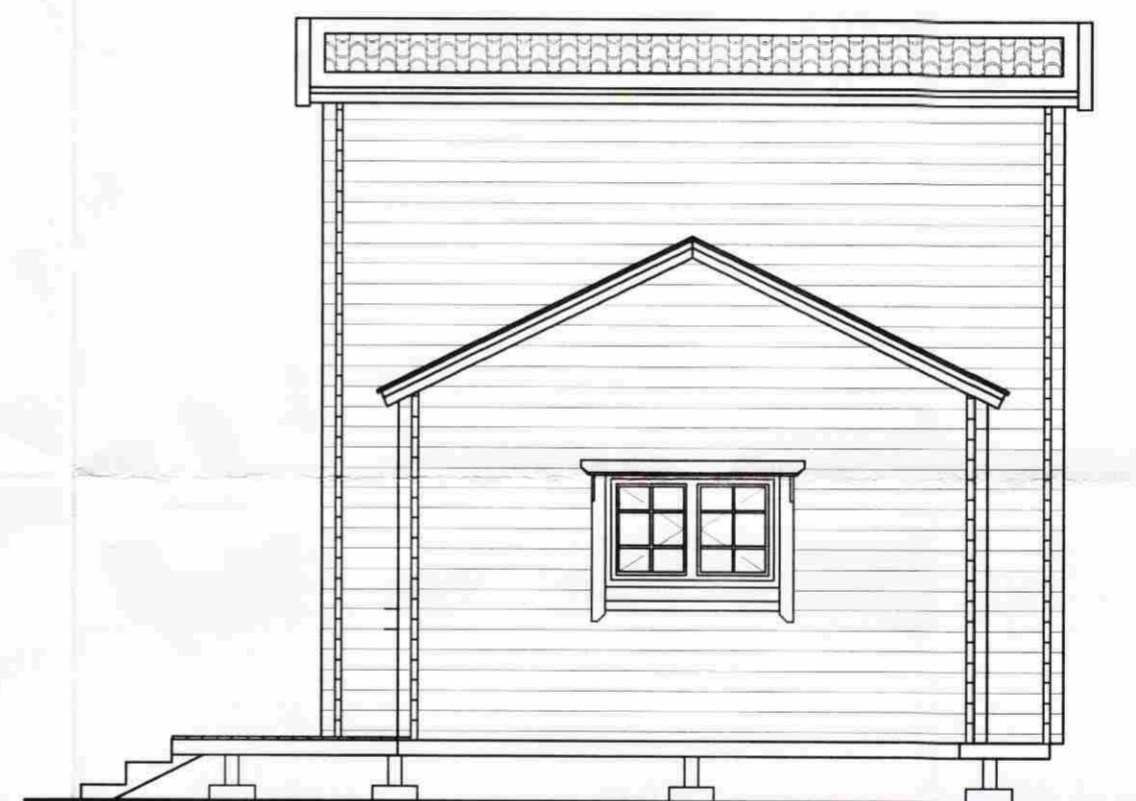
Austurhlíð 1:50
