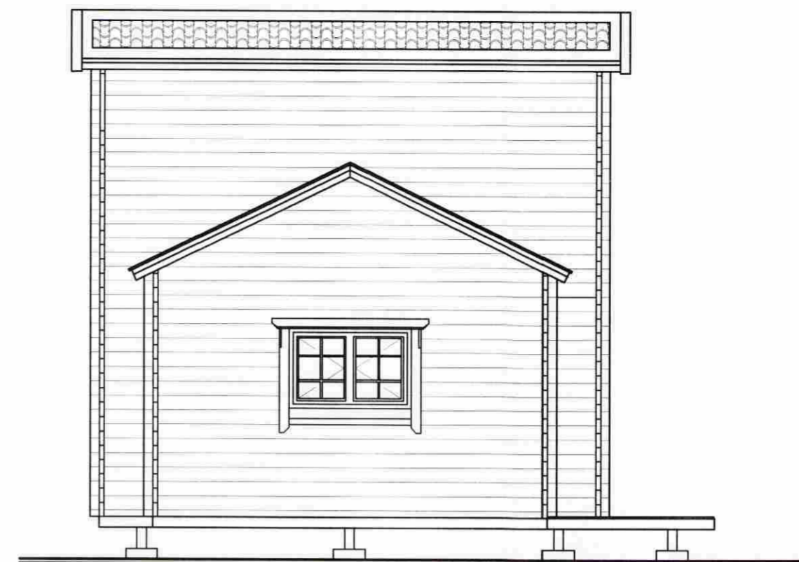
Vesturhlíð 1:50
