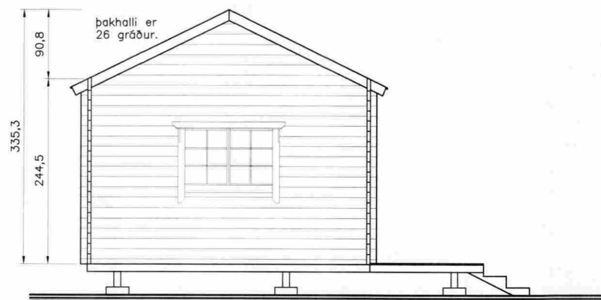
Sneiðing A 1:50
