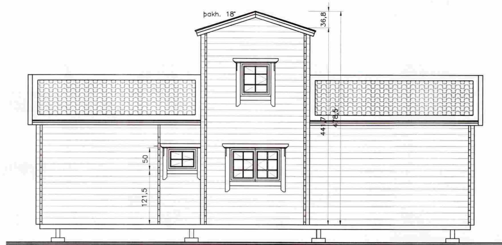
Norðurhlíð 1:50
