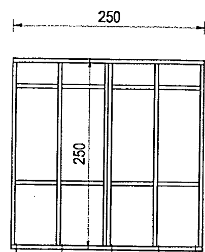
TENGIBYGGING TIMBURGRIND VESTUR HLIÐAR
