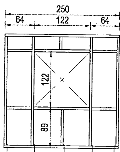
TENGIBYGGING TIMBURGRIND AUSTUR HLIÐAR
