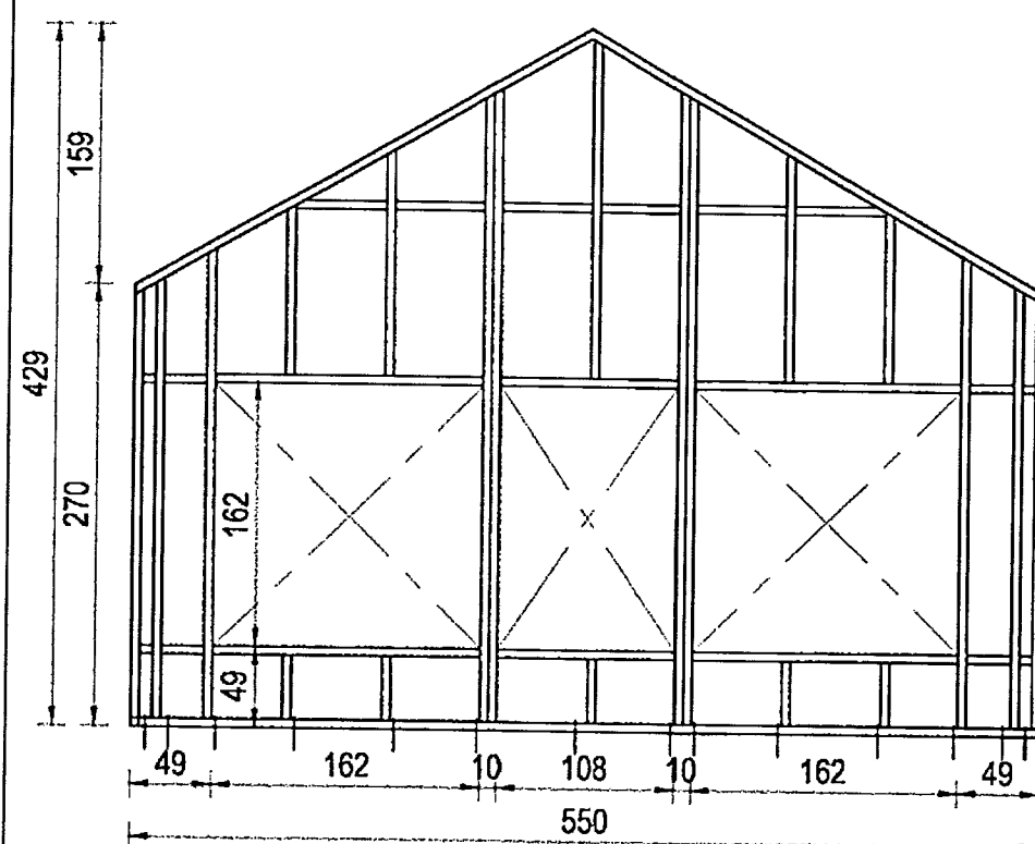
HÚS C, TIMBURGRIND AUSTUR HLIÐAR
