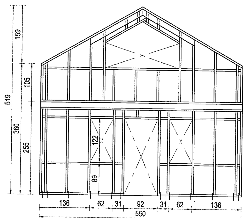
HÚS C, TIMBURGRIND AUSTUR HLIÐAR
