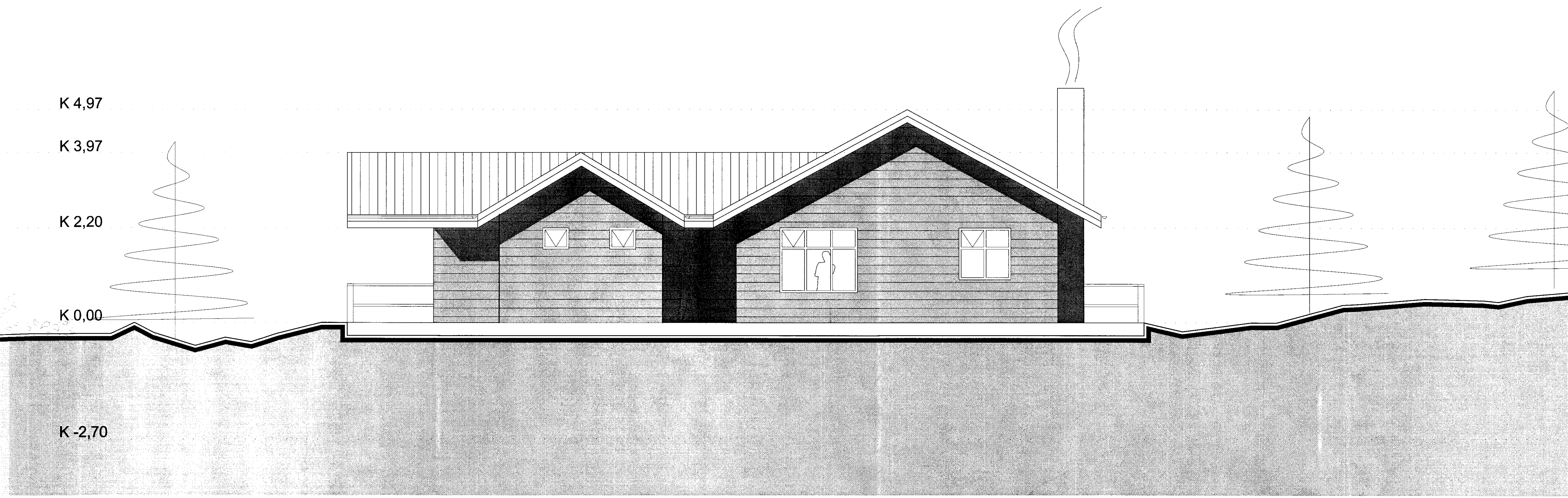
Útlit norður mkv. 1:50
