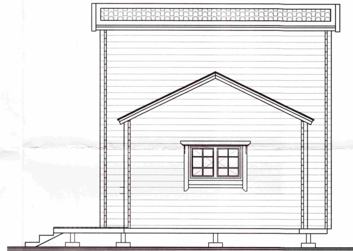
Austurhlíð 1:50
