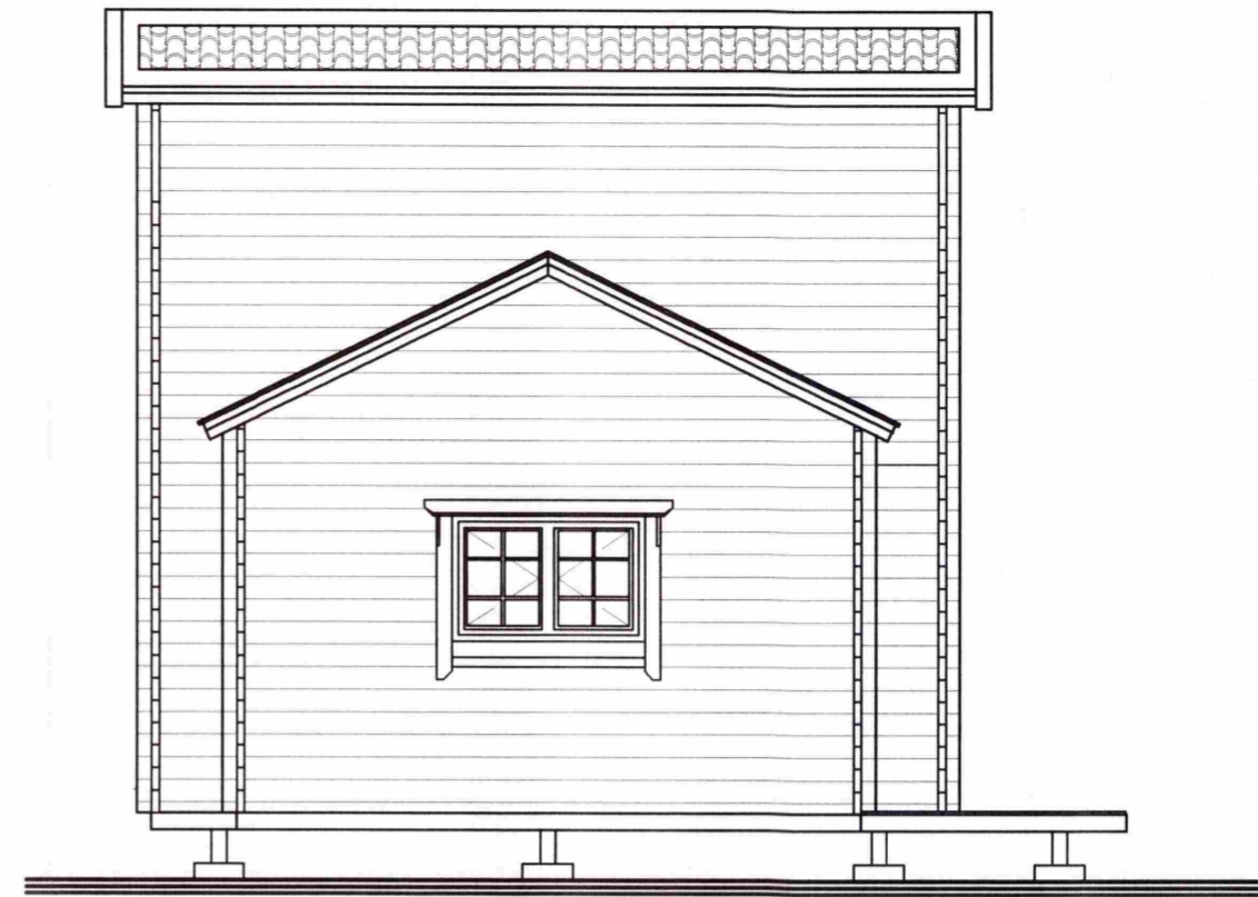
Vesturhlíð 1:50
