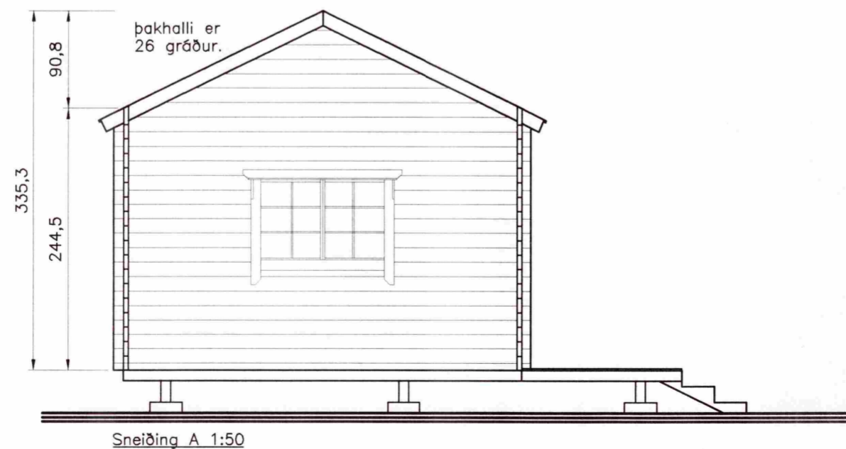
Sneiðing A 1:50
