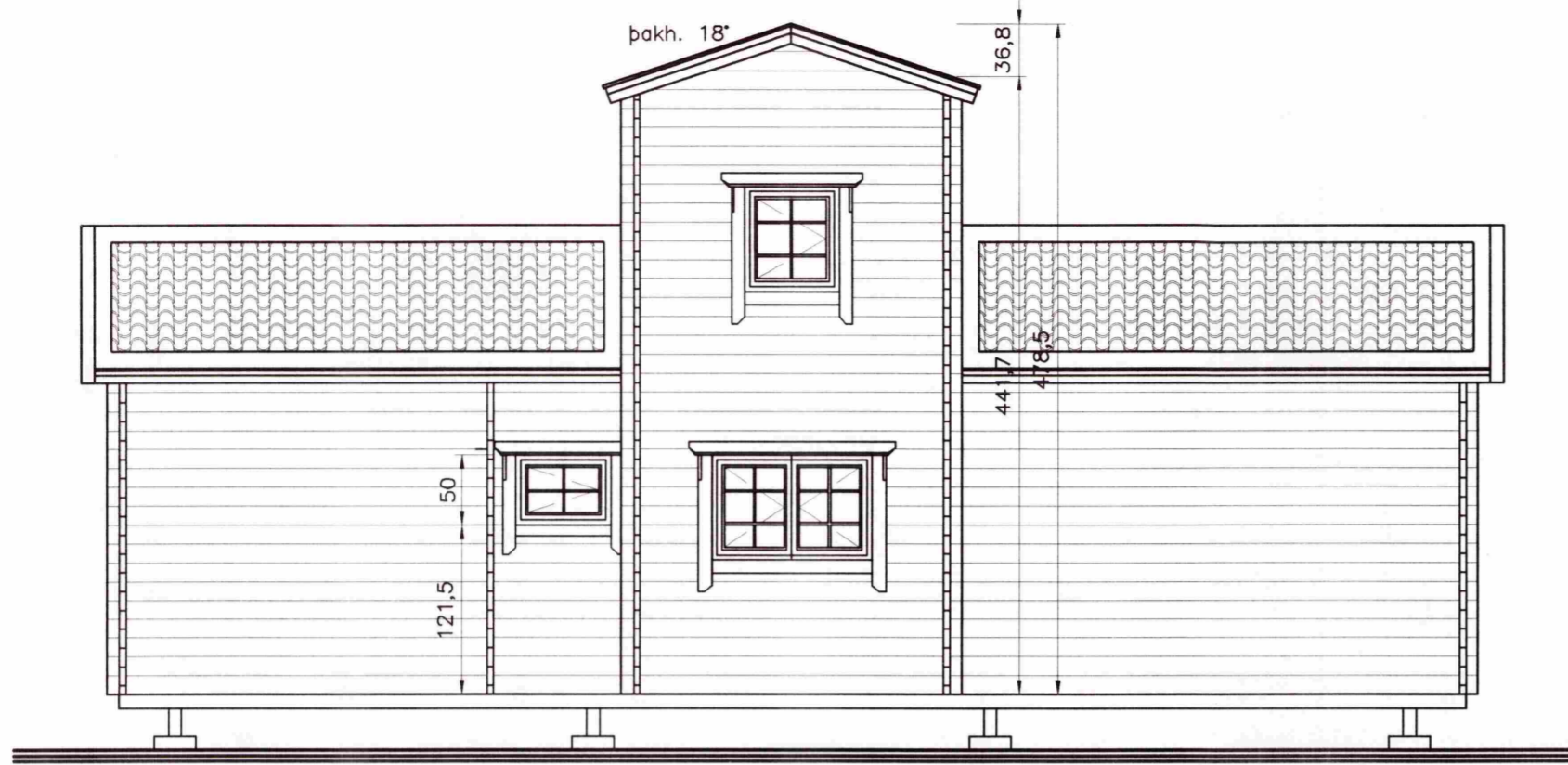
Norðurhlíð 1:50
